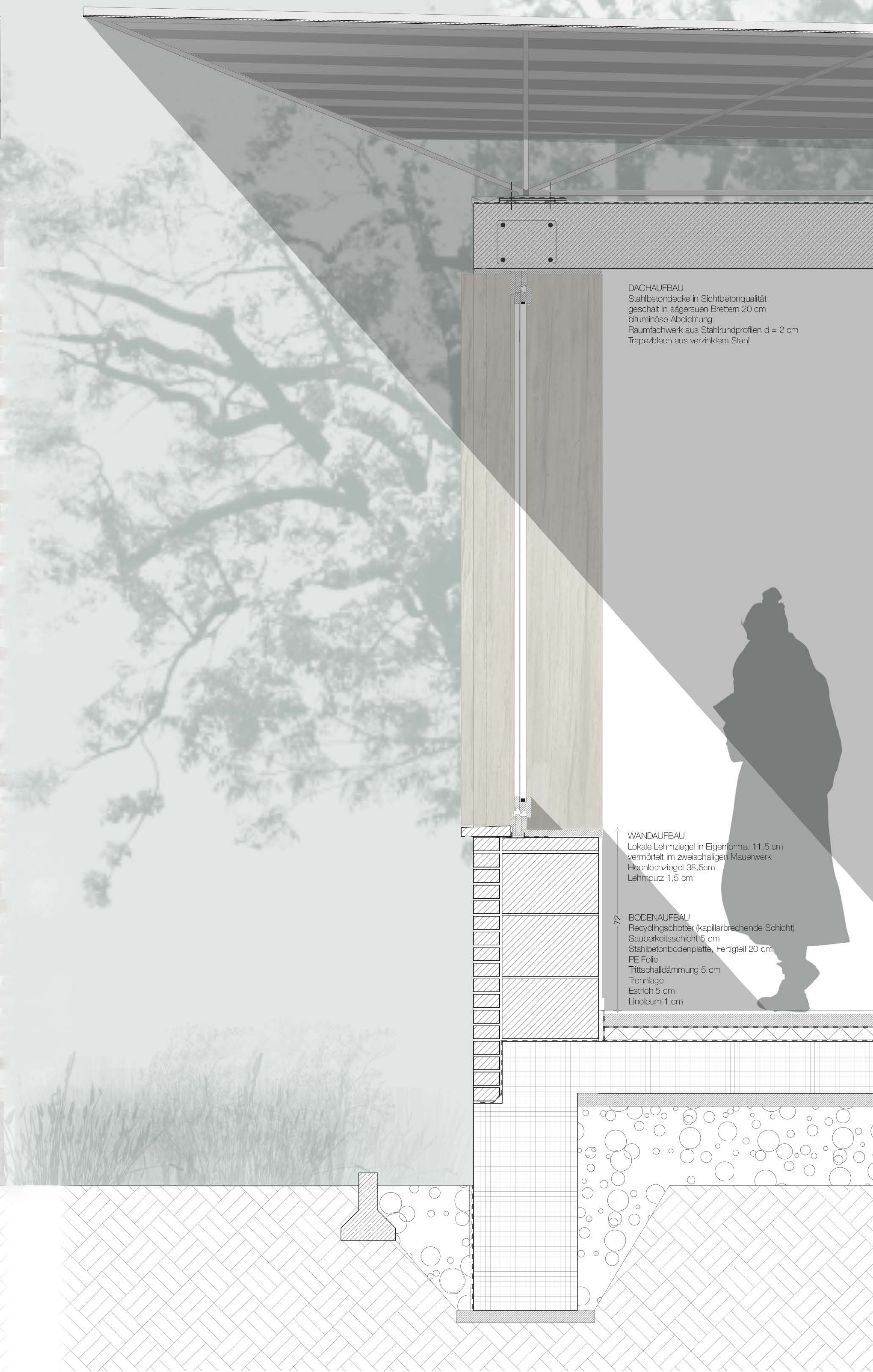
FASSADENSCHNITT_M 1.10
