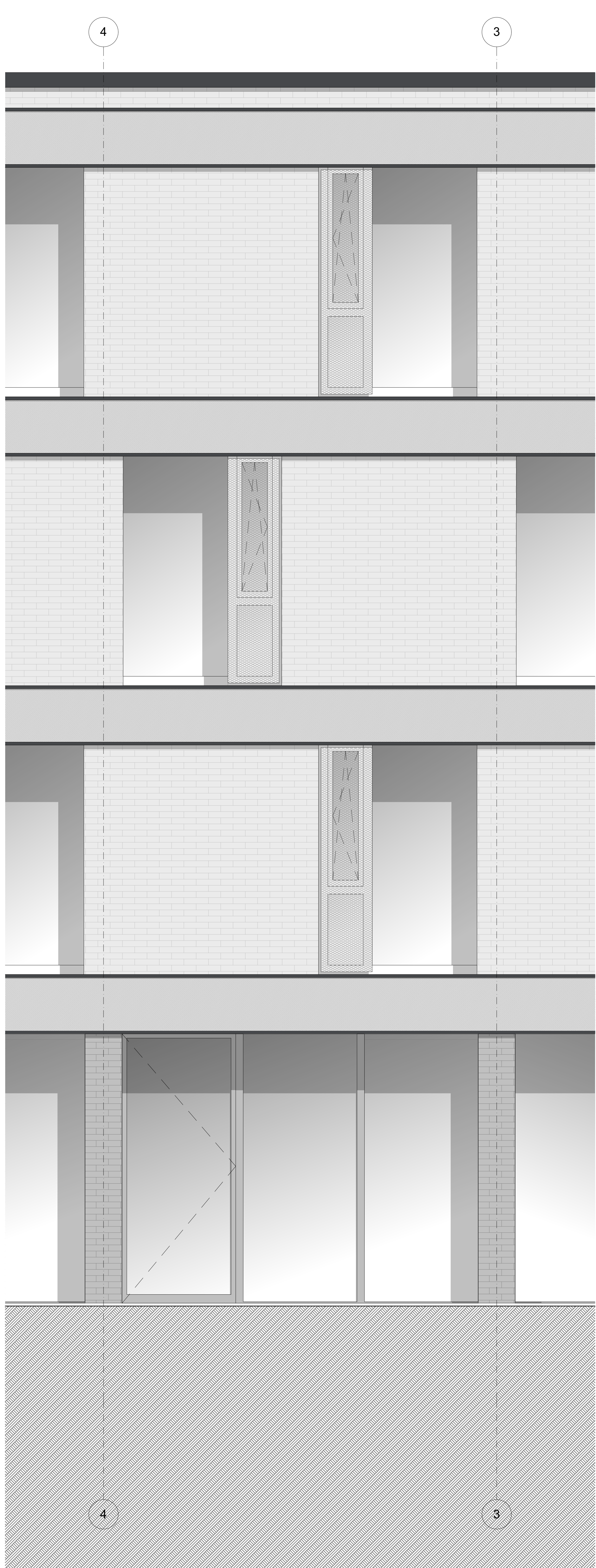
ANSICHT NORD
