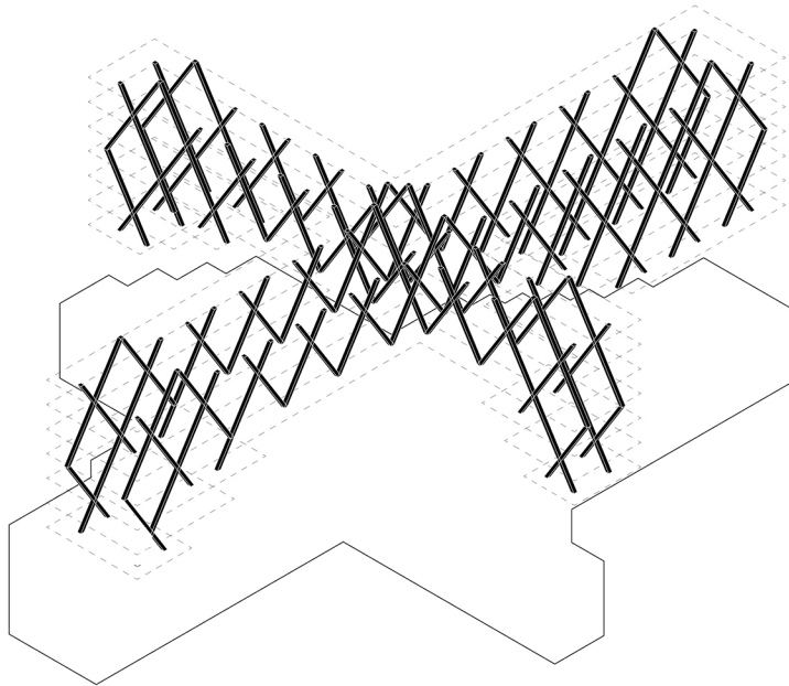
3. Das geschossübergreifende Tragwerk mit aussteifenden Diagonalstäben
