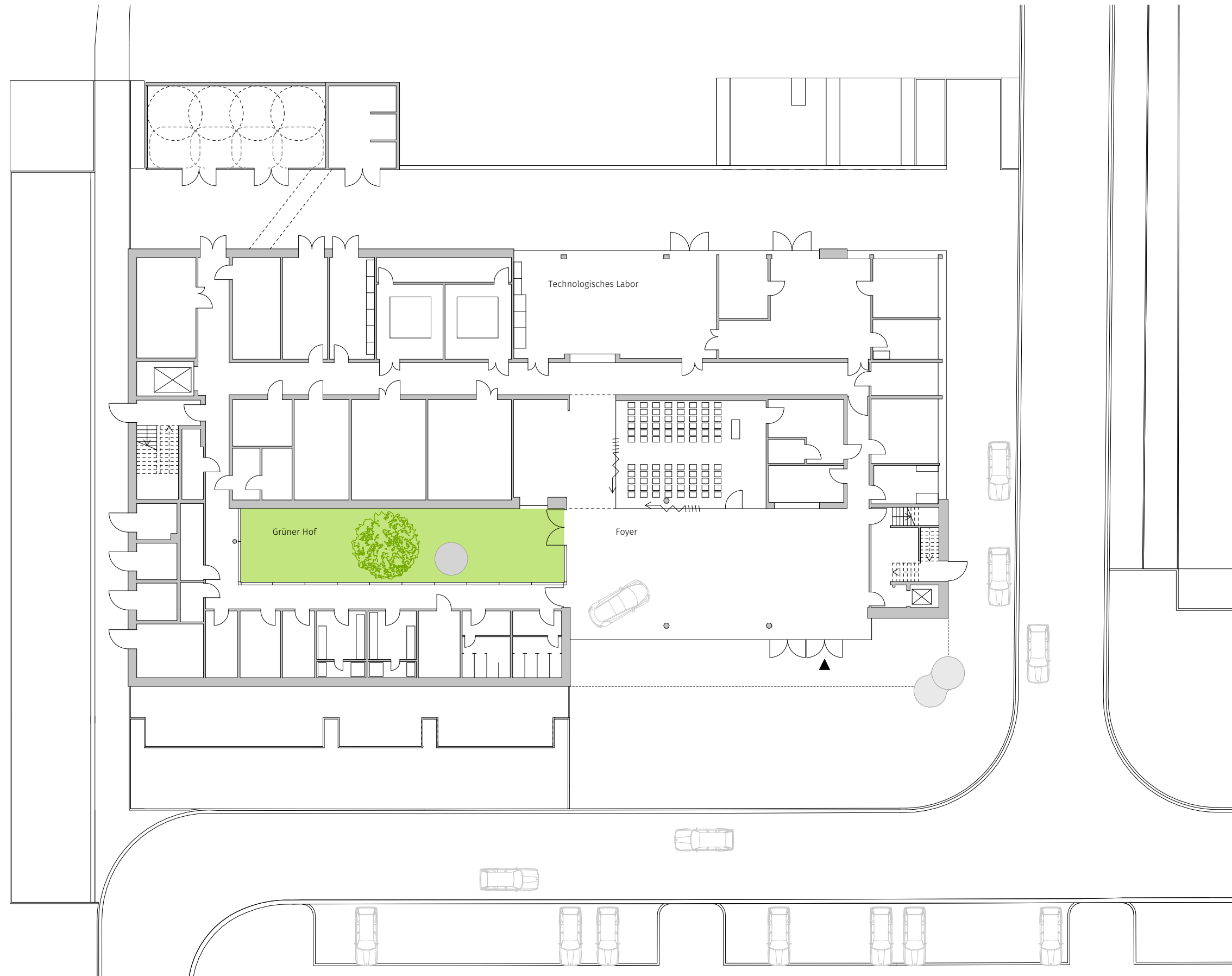
Grundriss Erdgeschoss M1:300
