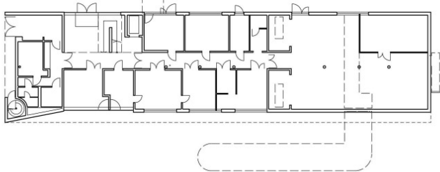
Grundriss E0
