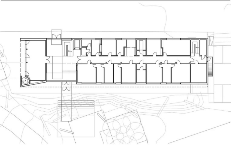
Grundriss E1
