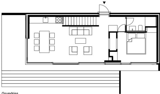
Grundriss Erdgeschoss
