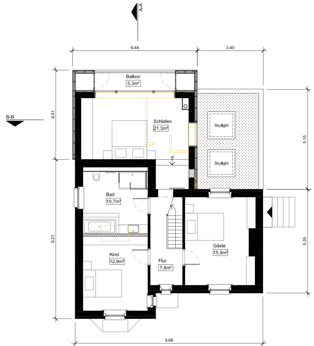
GRUNDRISS OBERGESCHOSS nach dem Umbau
