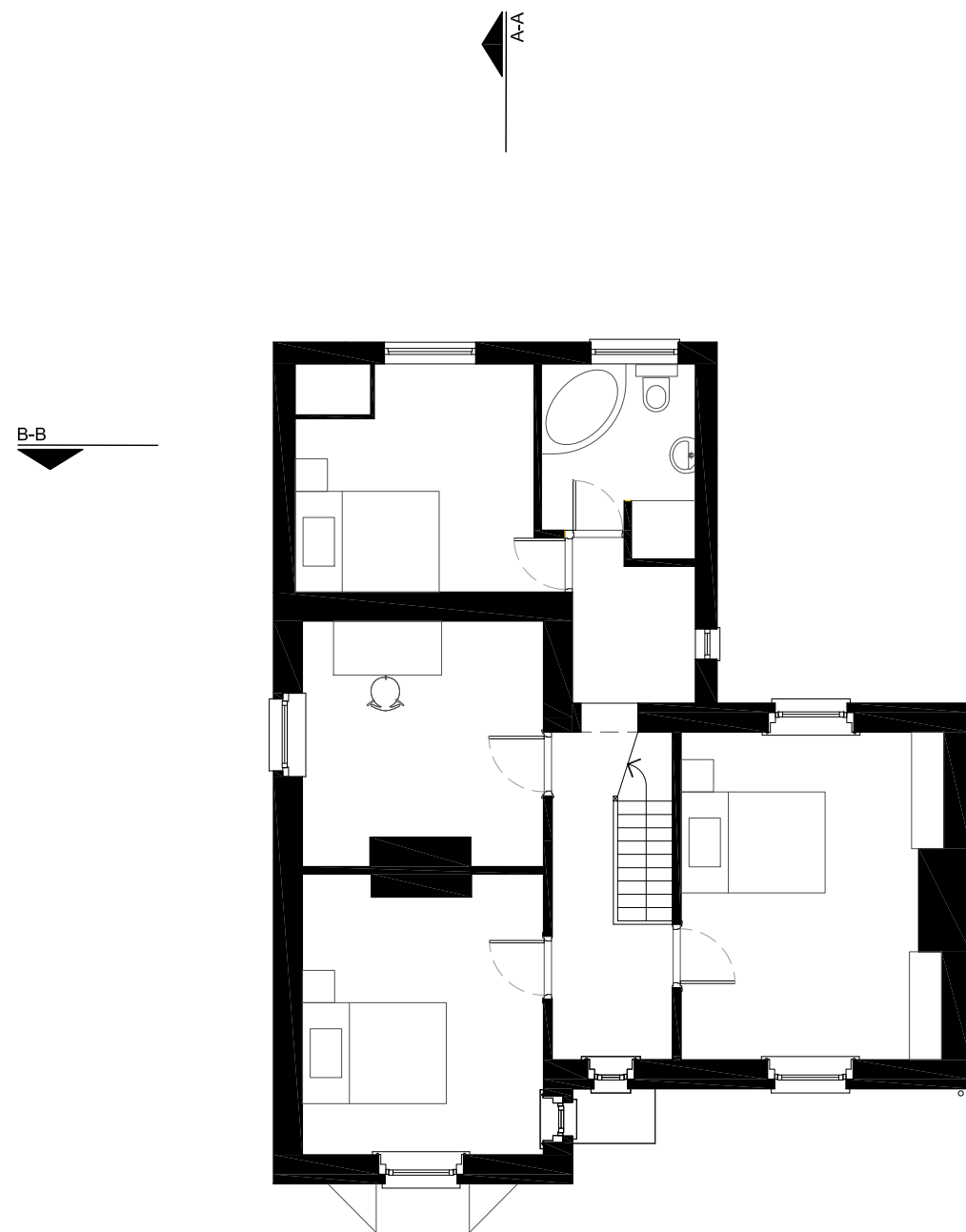
GRUNDRISS OBERGESCHOSS Bestand
