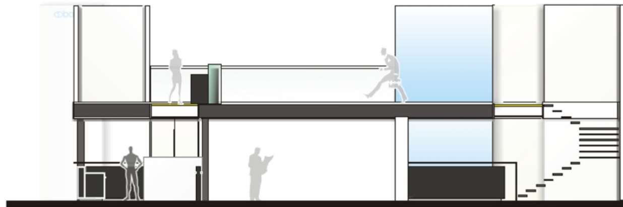
Schnitt B-B
