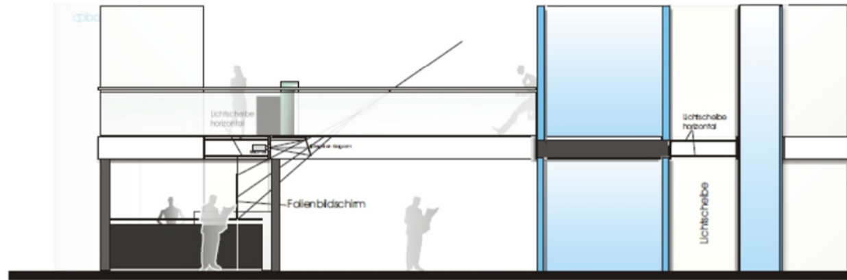
Schnitt C-C
