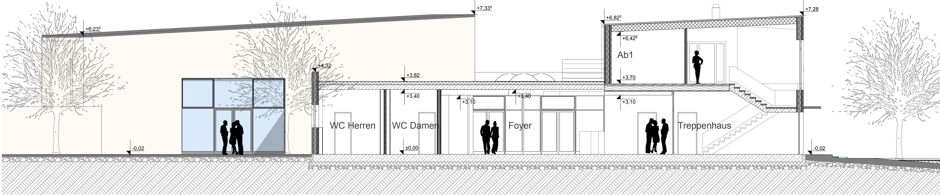
Schnitt a-a
