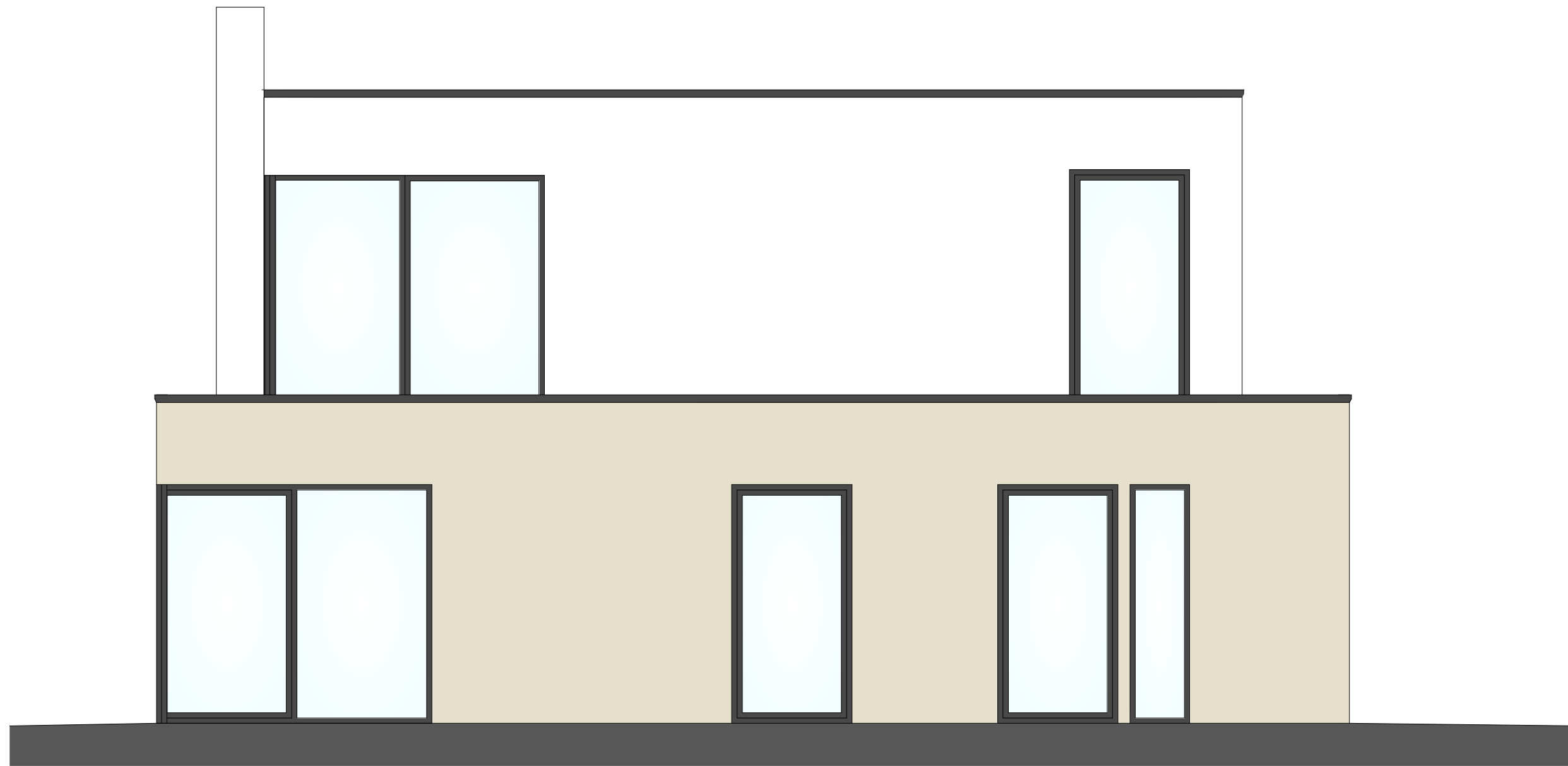
Südansicht (Garten)
