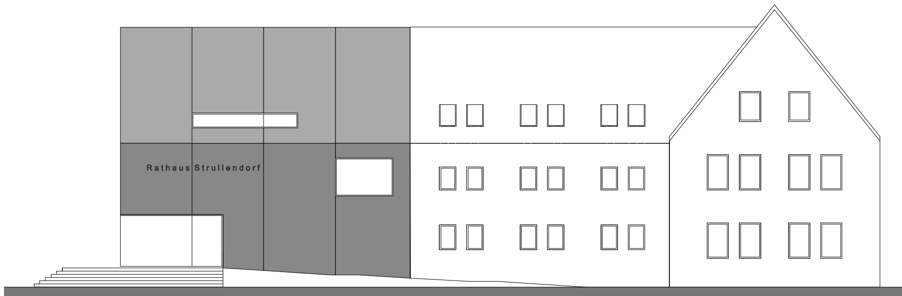
Ansicht Süd-West
