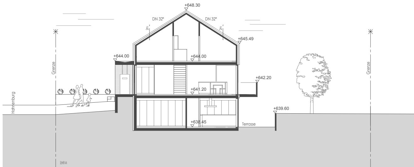
sCHNITT A-A 1_200
