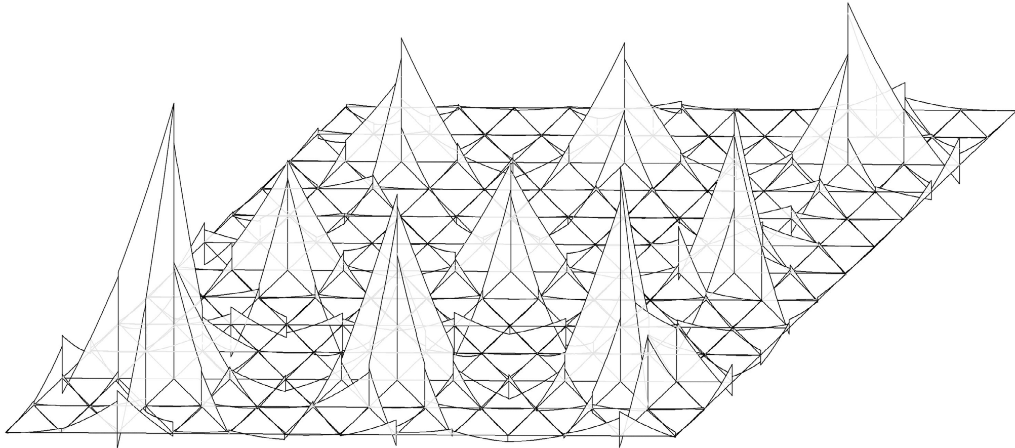
Momentenverläufe höchstes Moment: 2196kNm
