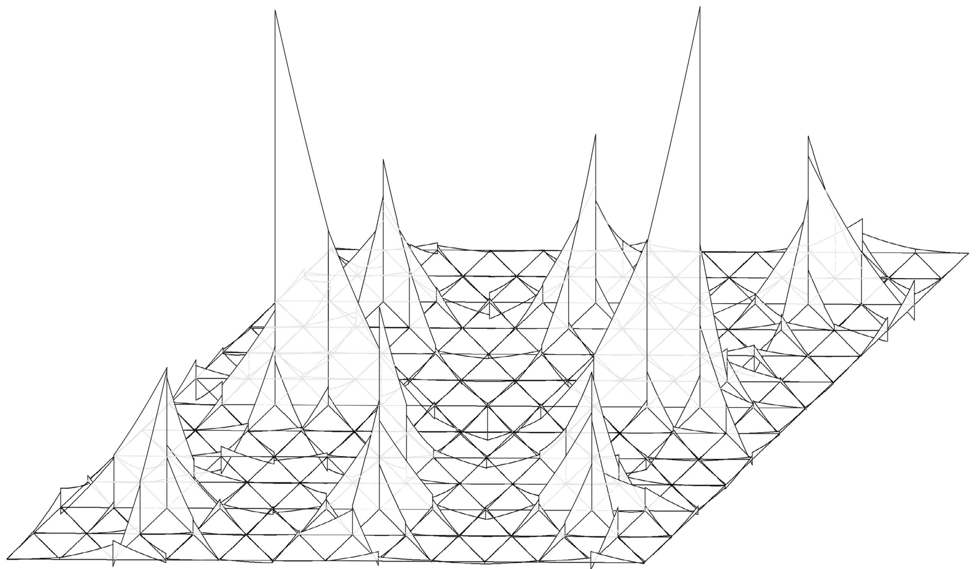
Momentenverläufe höchstes Moment: 4109kNm
