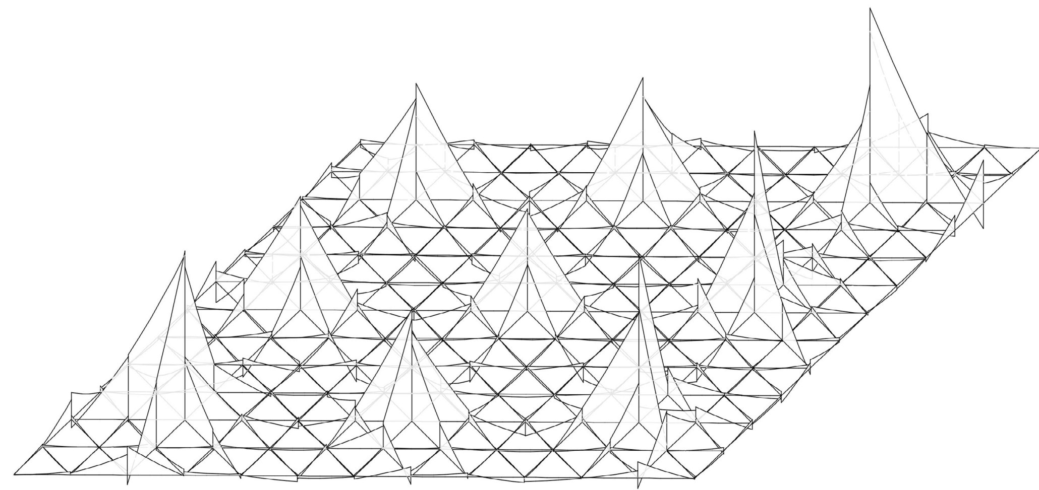
Momentenverläufe höchstes Moment: 1963kNm
