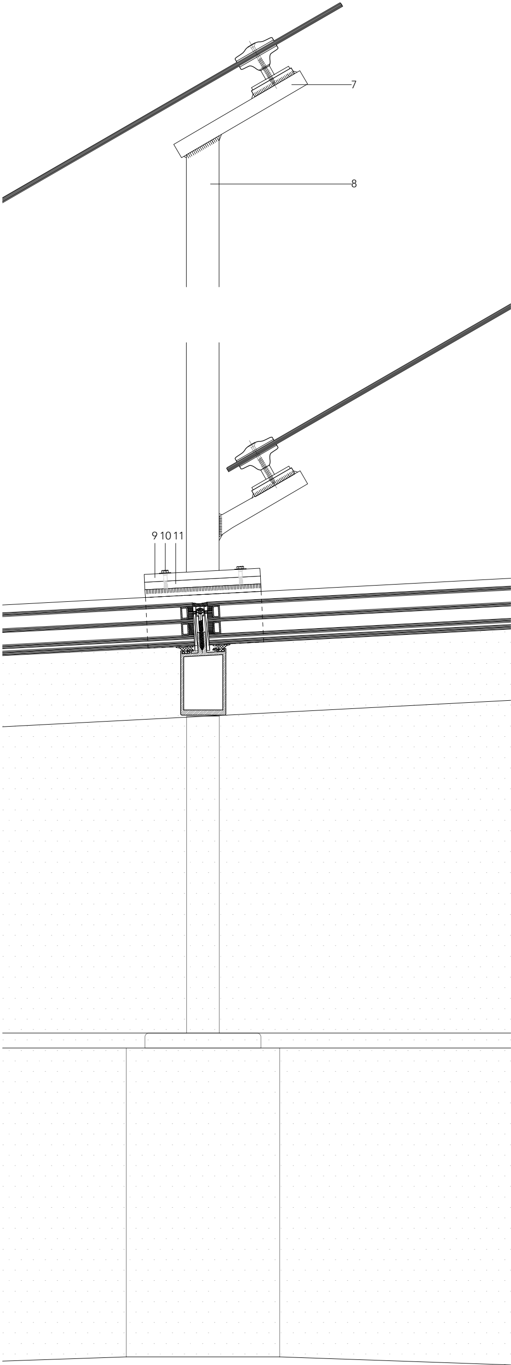
Detail Oberlicht M_1:5
