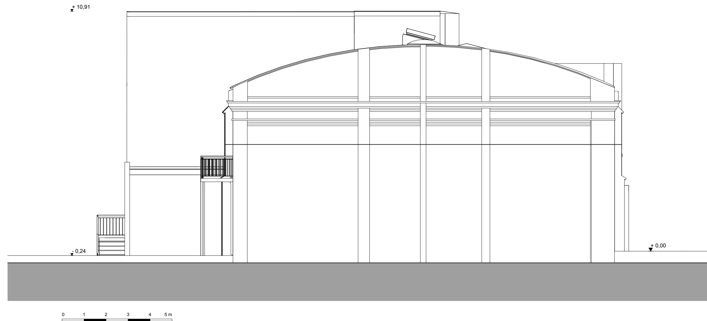
Ansicht Nord
