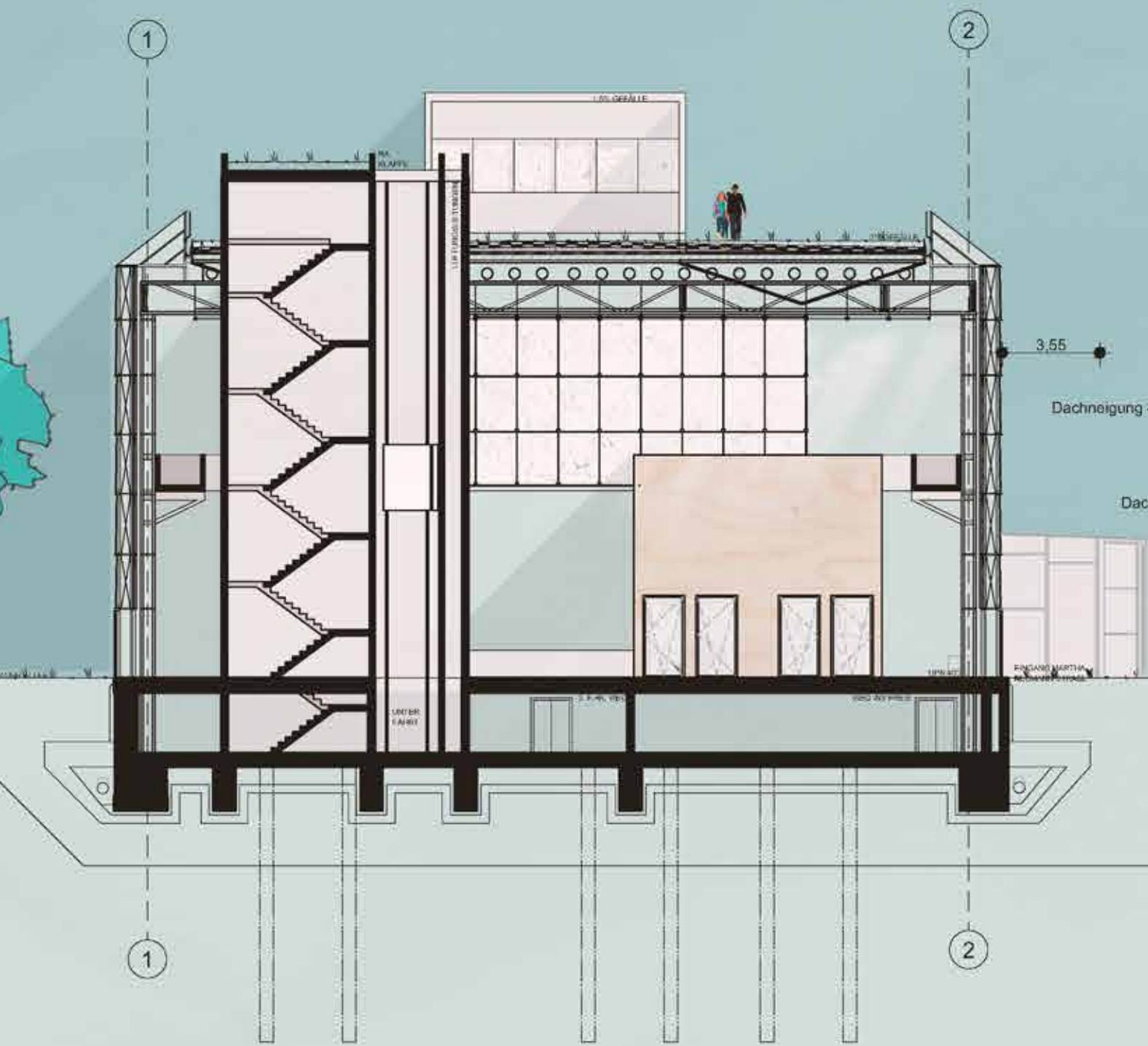
SCHNITT CC
