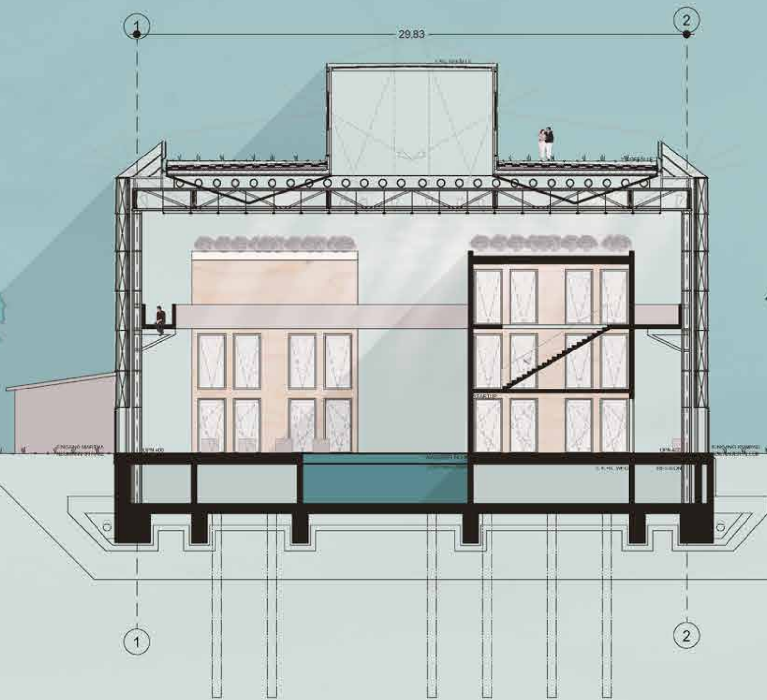
SCHNITT BB
