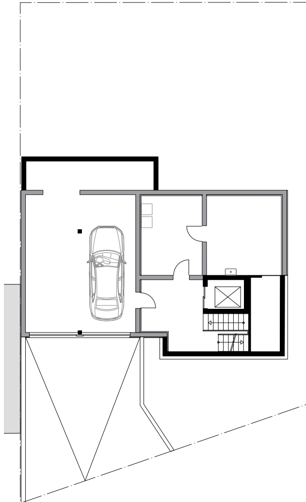
Grundriss UG M 1:200
