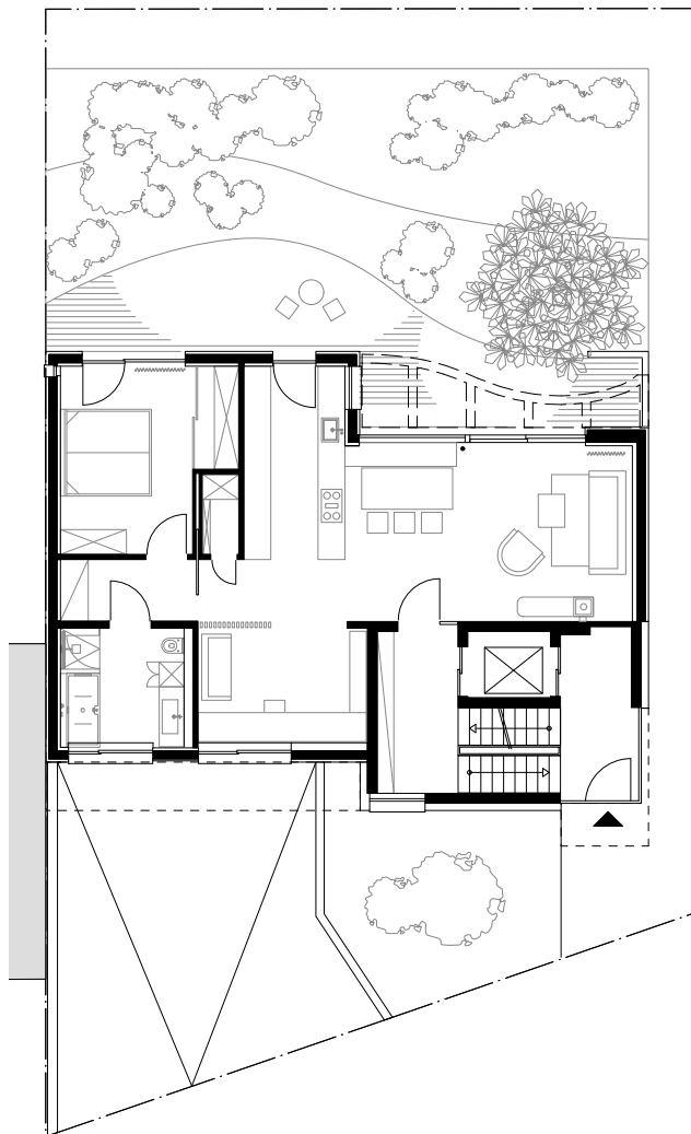
Grundriss EG M 1:200
