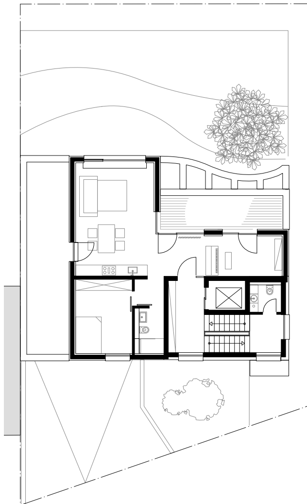
Grundriss DG M 1:200
