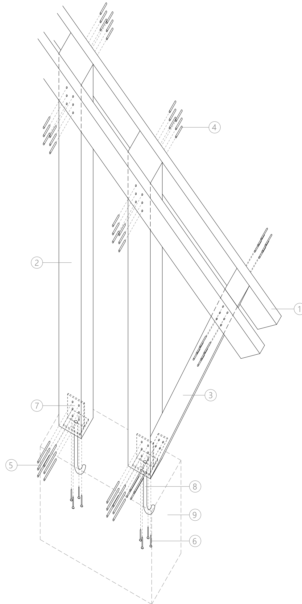
Konstruktiver Knoten
