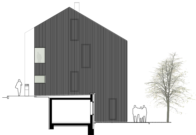
Westansicht
