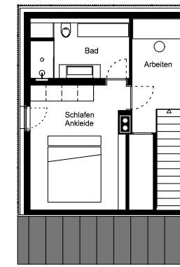
Dachgeschoss
