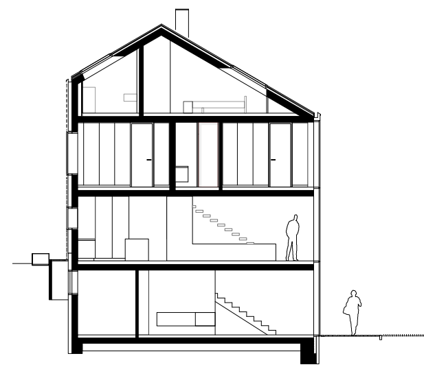
Schnitt
