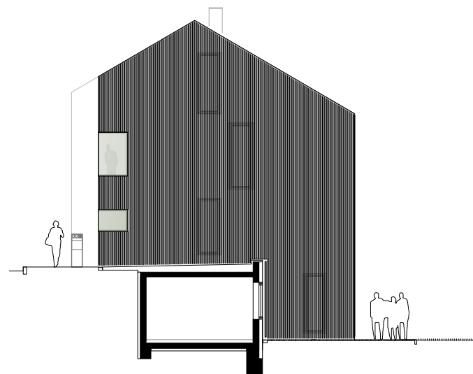
Westansicht
