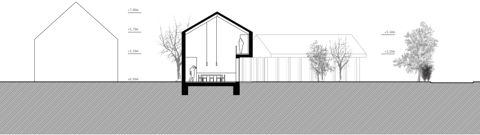
Schnitt AA 1:250
