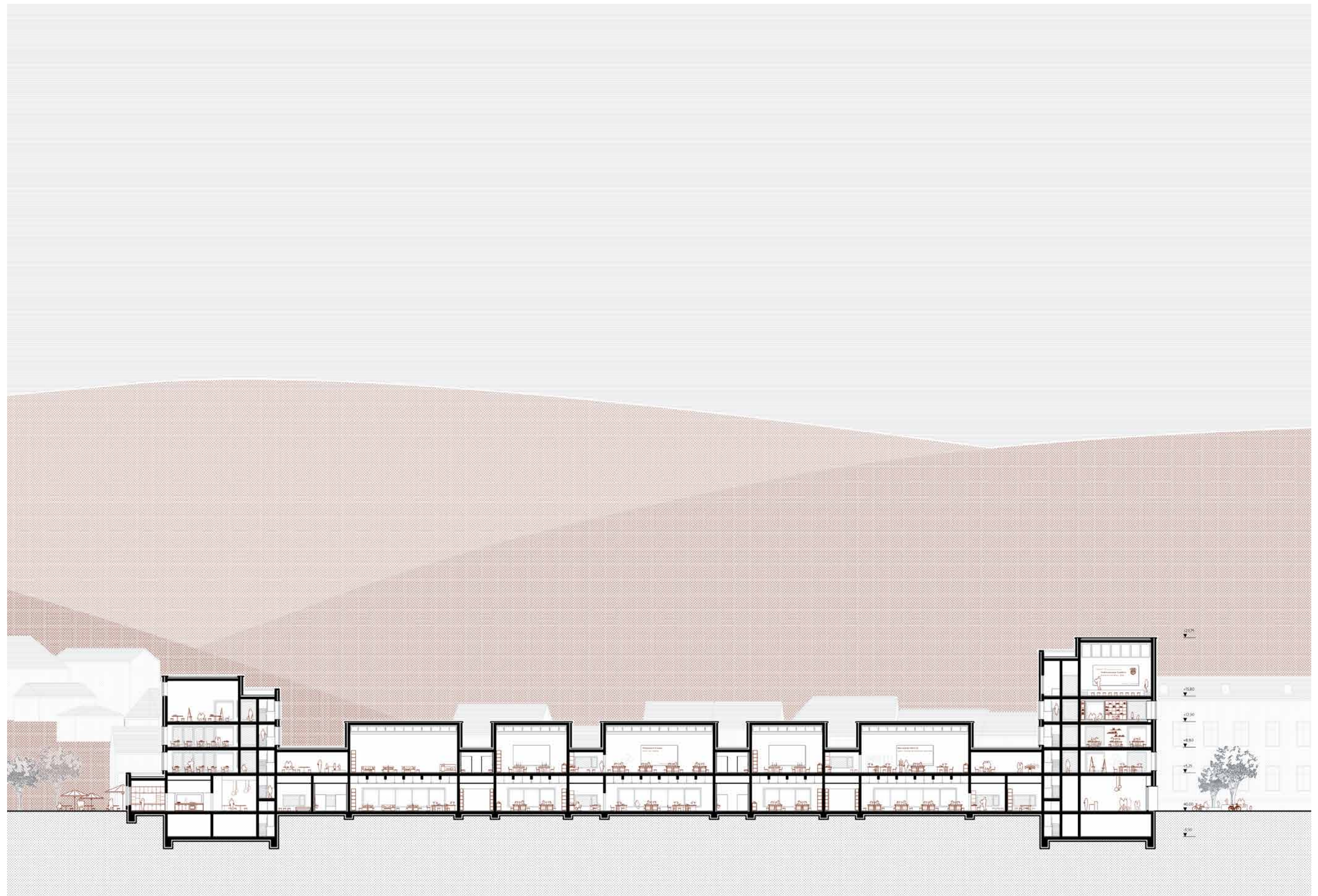
LÄNGSSCHNITT A-A
