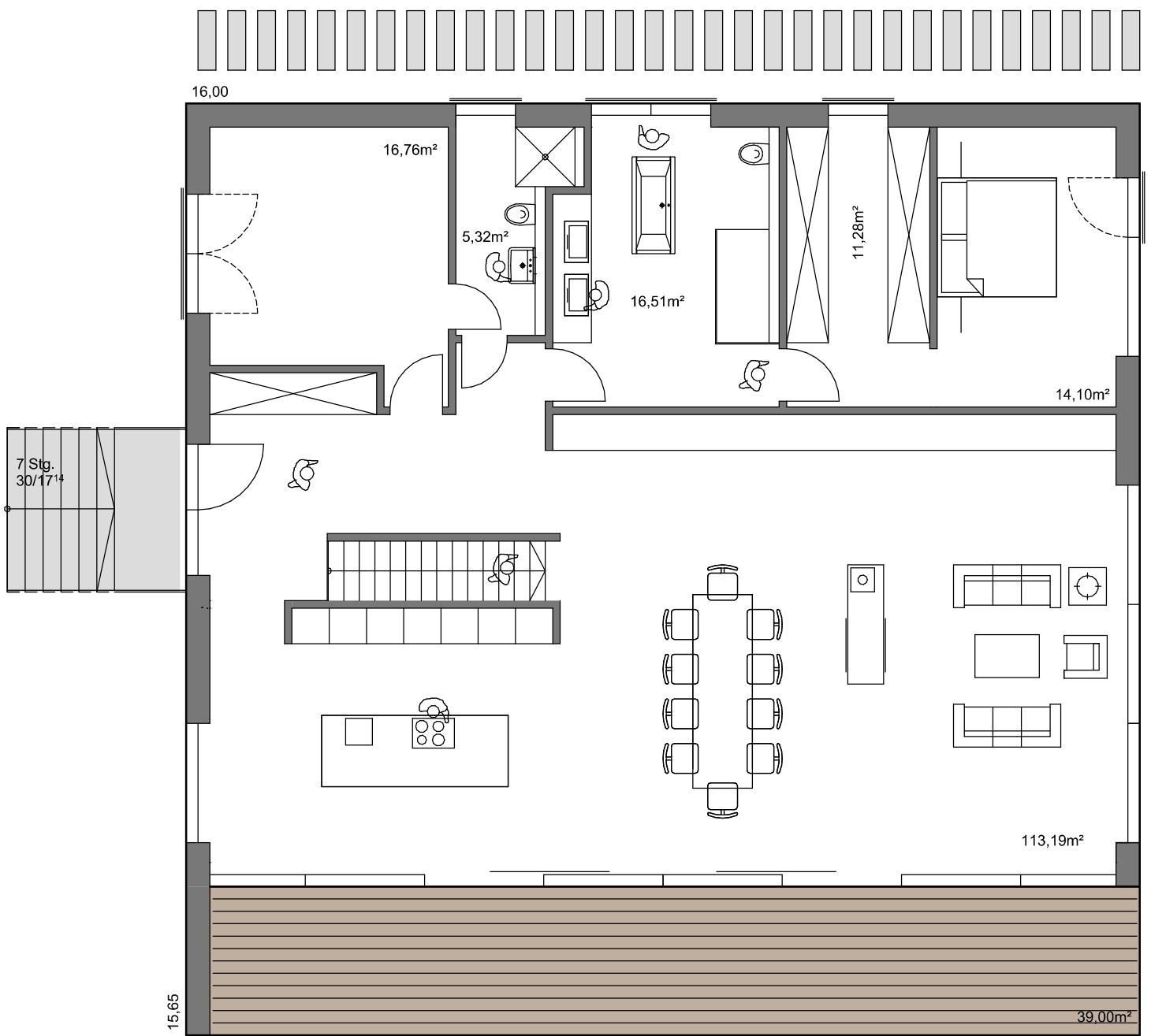
Grundriss Erdgeschoss
