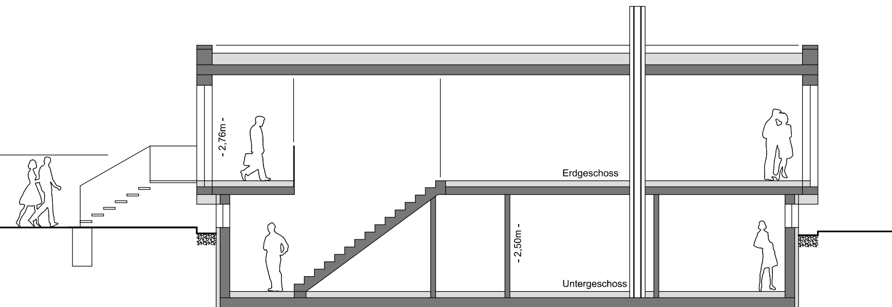
Gebäudeschnitt
