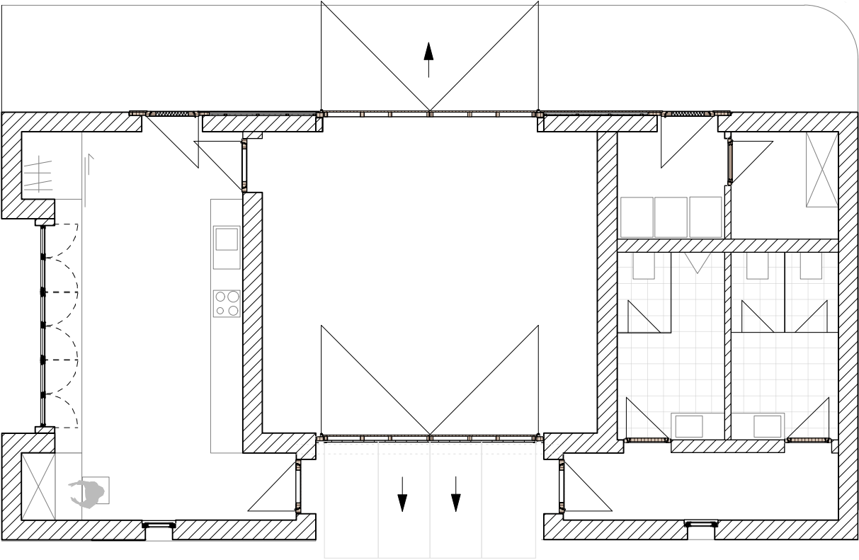
Grundriss M 1:100
