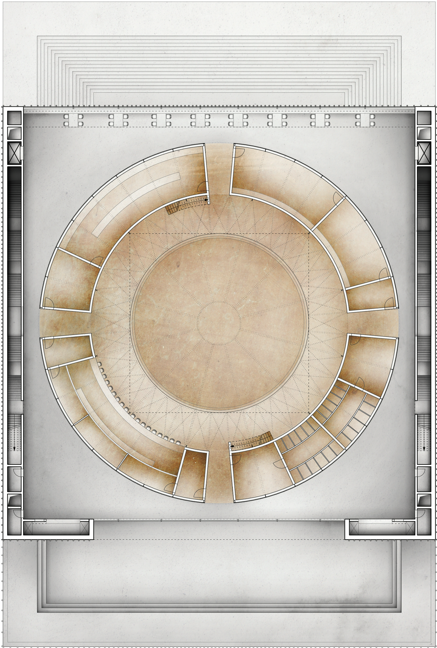
GRUNDRISS 2.OG 1:200
