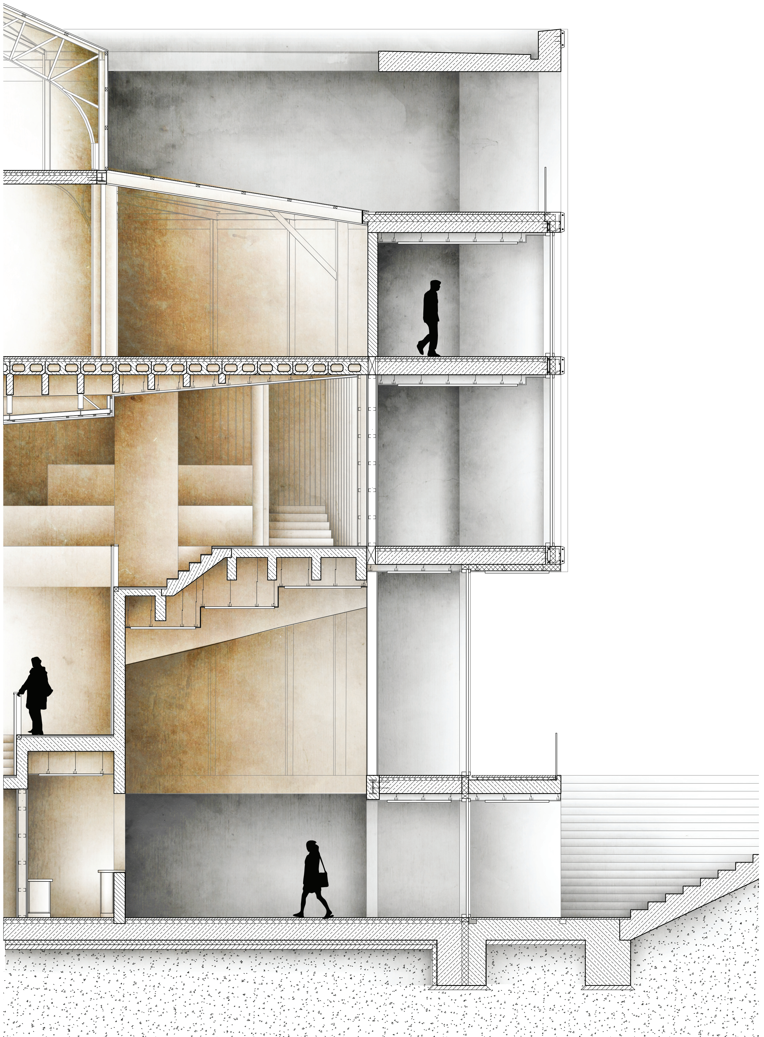
FASSADENSCHNITT 1:50
