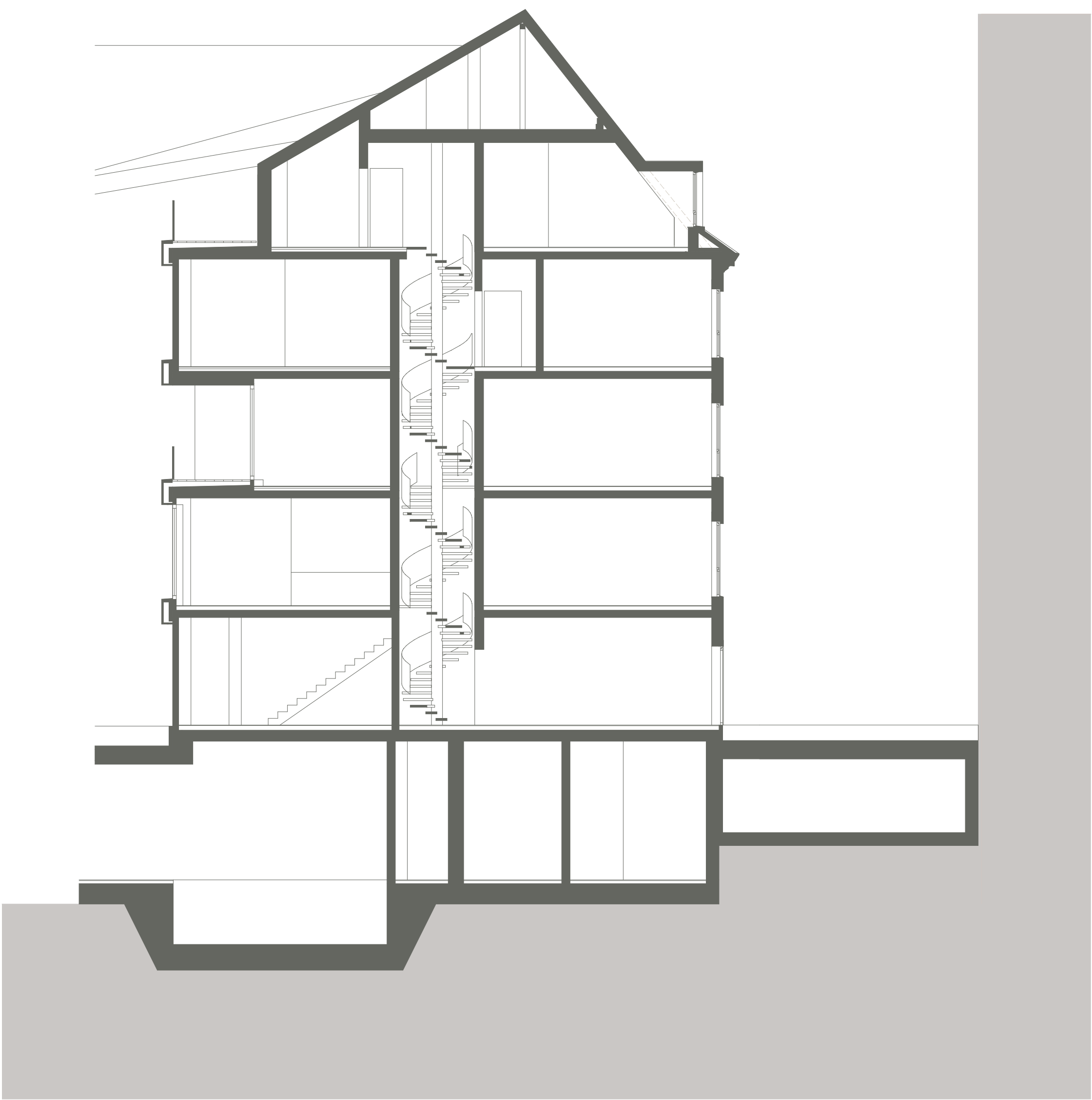
SCHNITT CC
