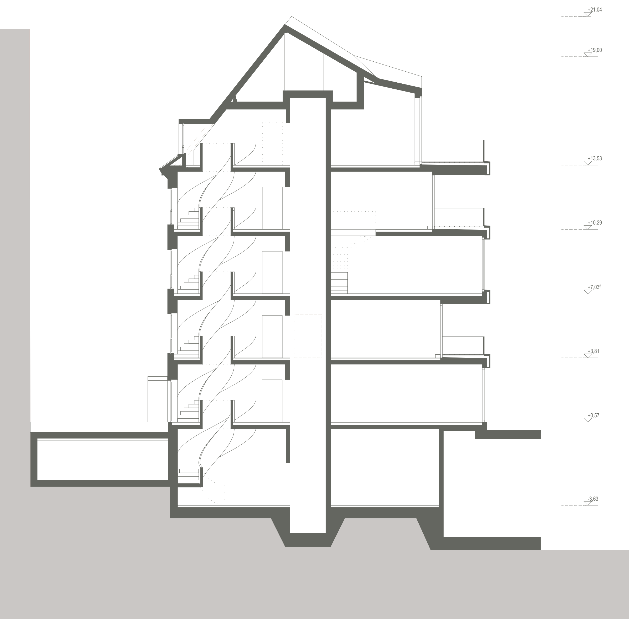
SCHNITT BB
