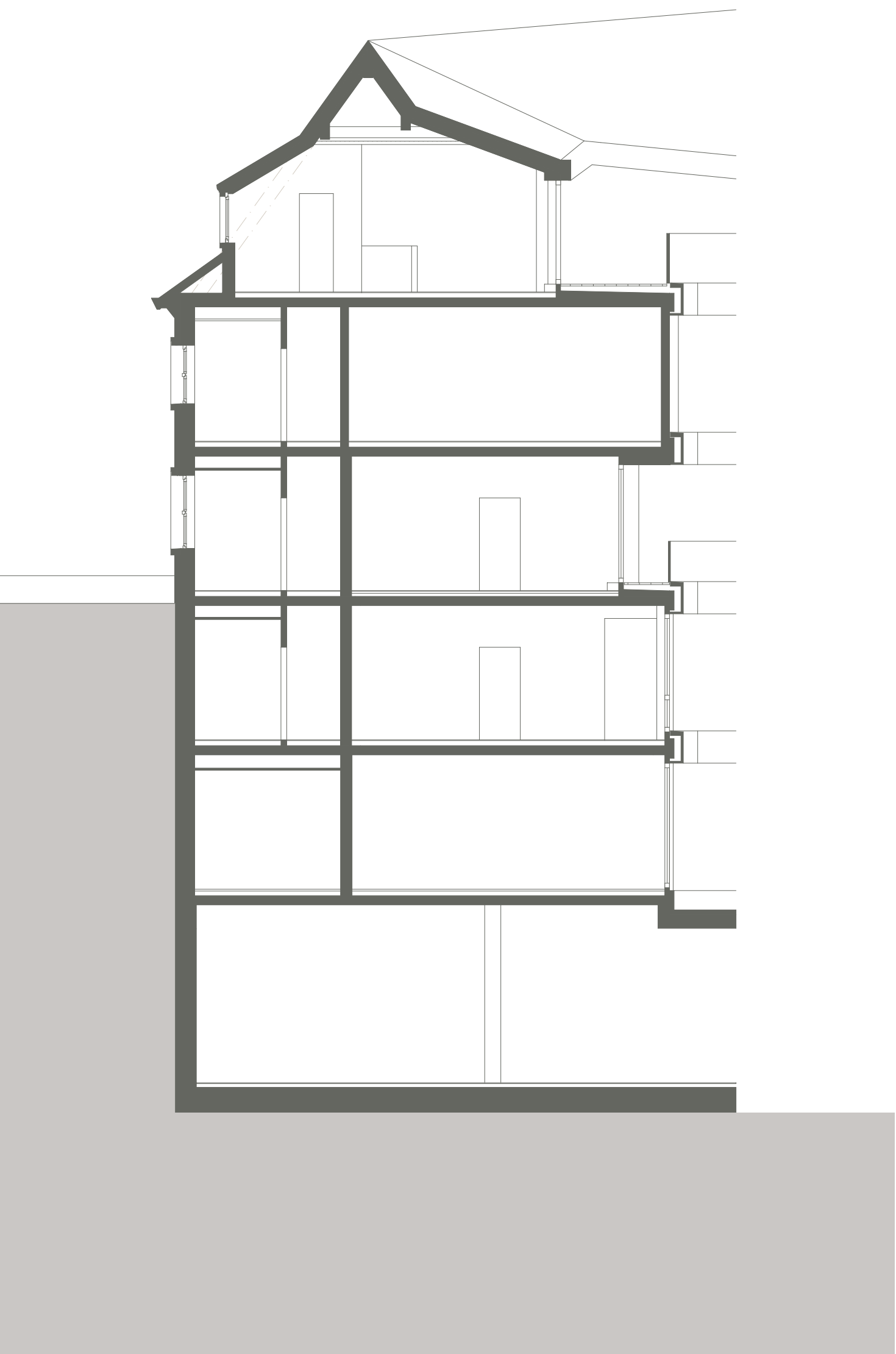
SCHNITT DD
