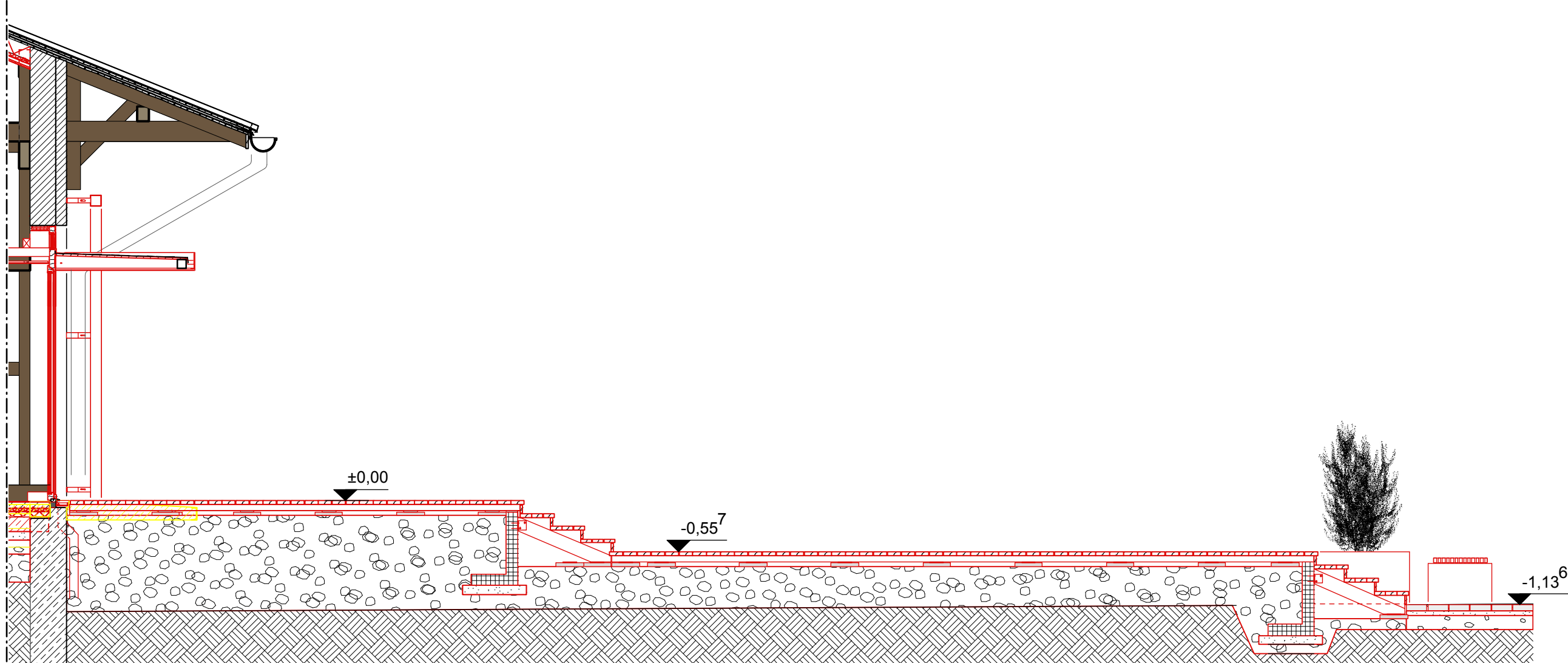
Geländeschnitt BB
