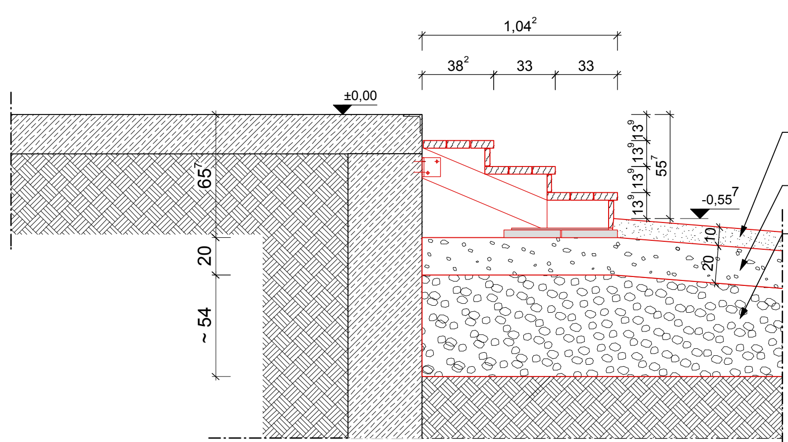
Geländeschnitt DD
