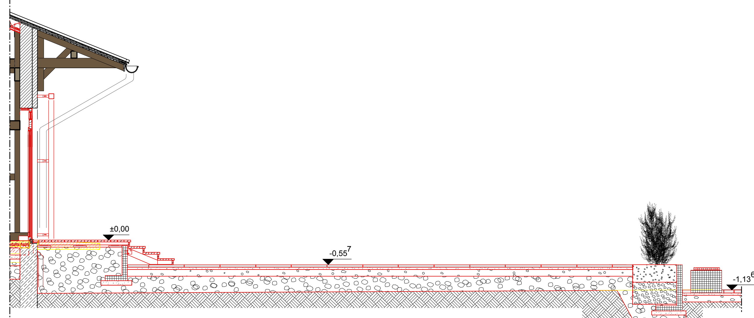
Geländeschnitt CC
