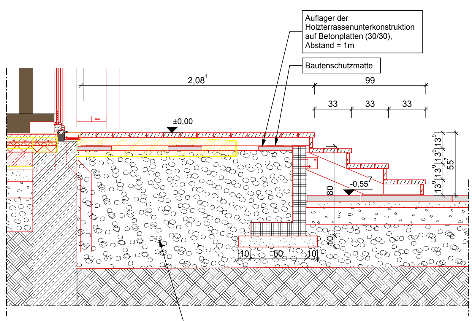
Geländeschnitt CC
