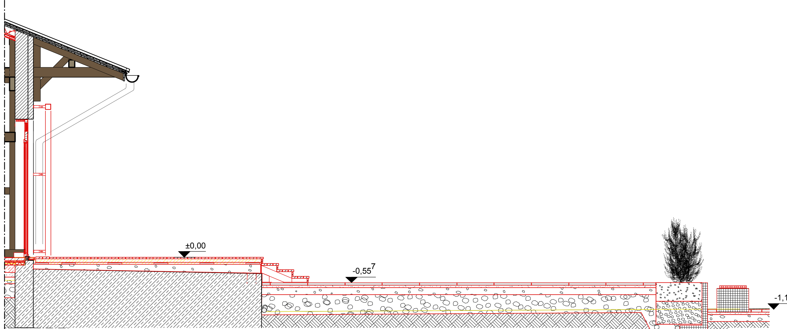
Geländeschnitt AA
