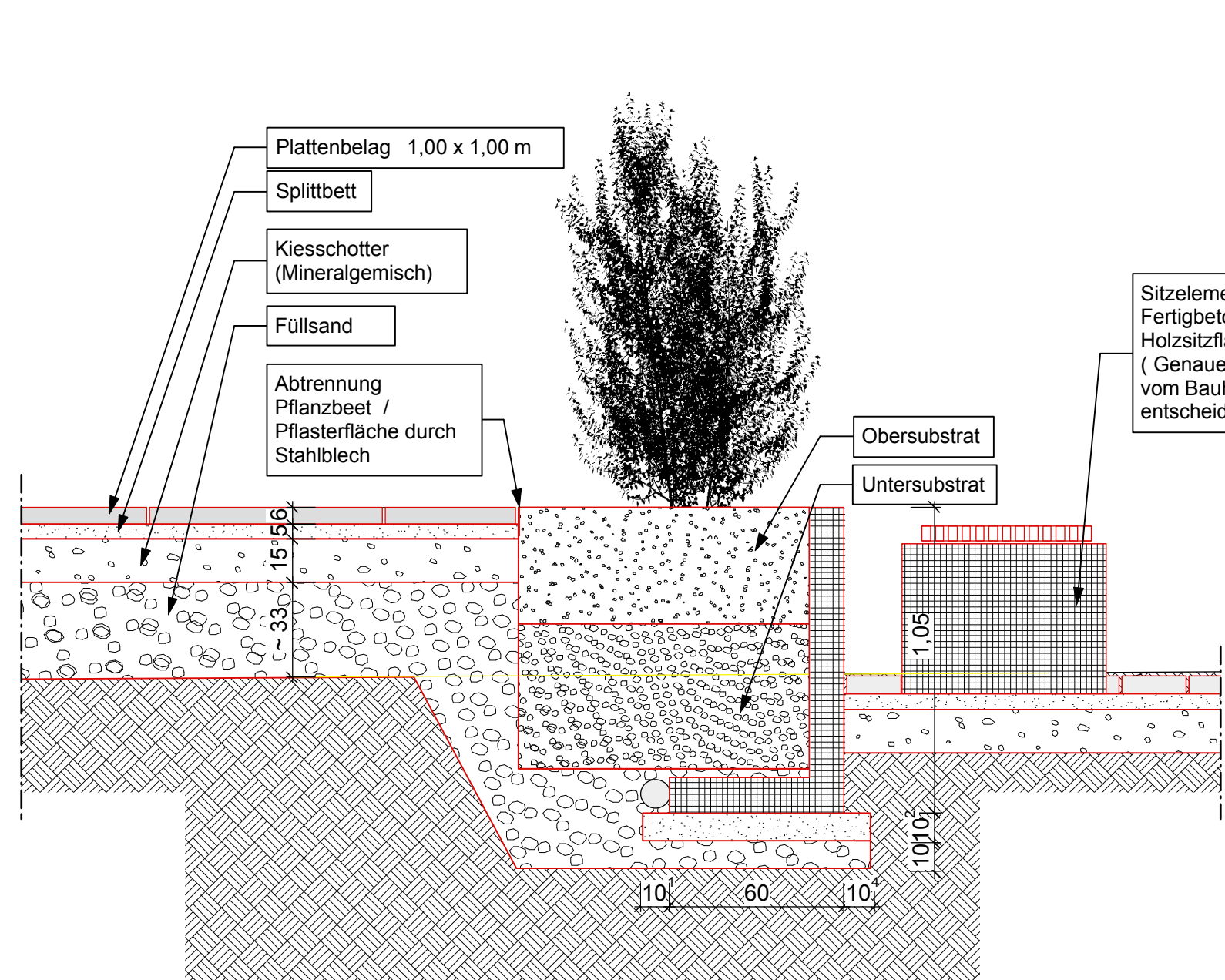
Detail Geländeschnitt CC M 1:20
