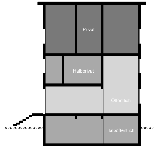
Schnitt B-B
