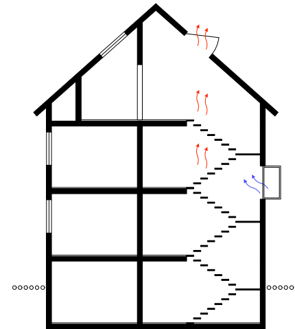
Schnitt C-C
