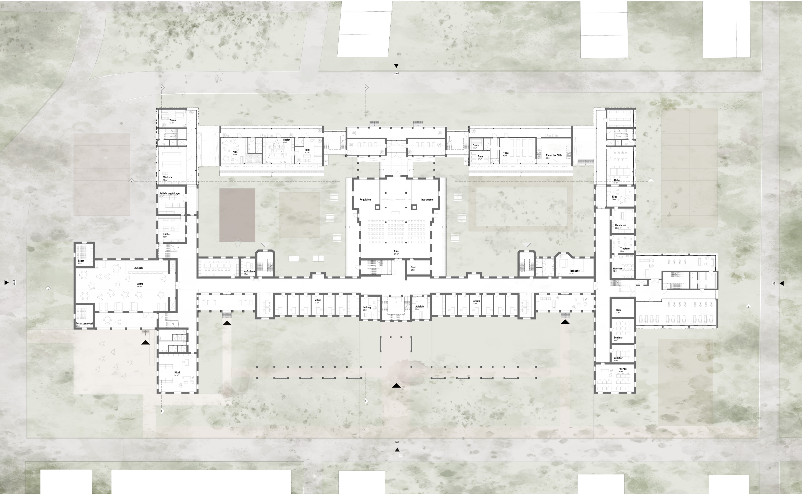
Grundriss EG
