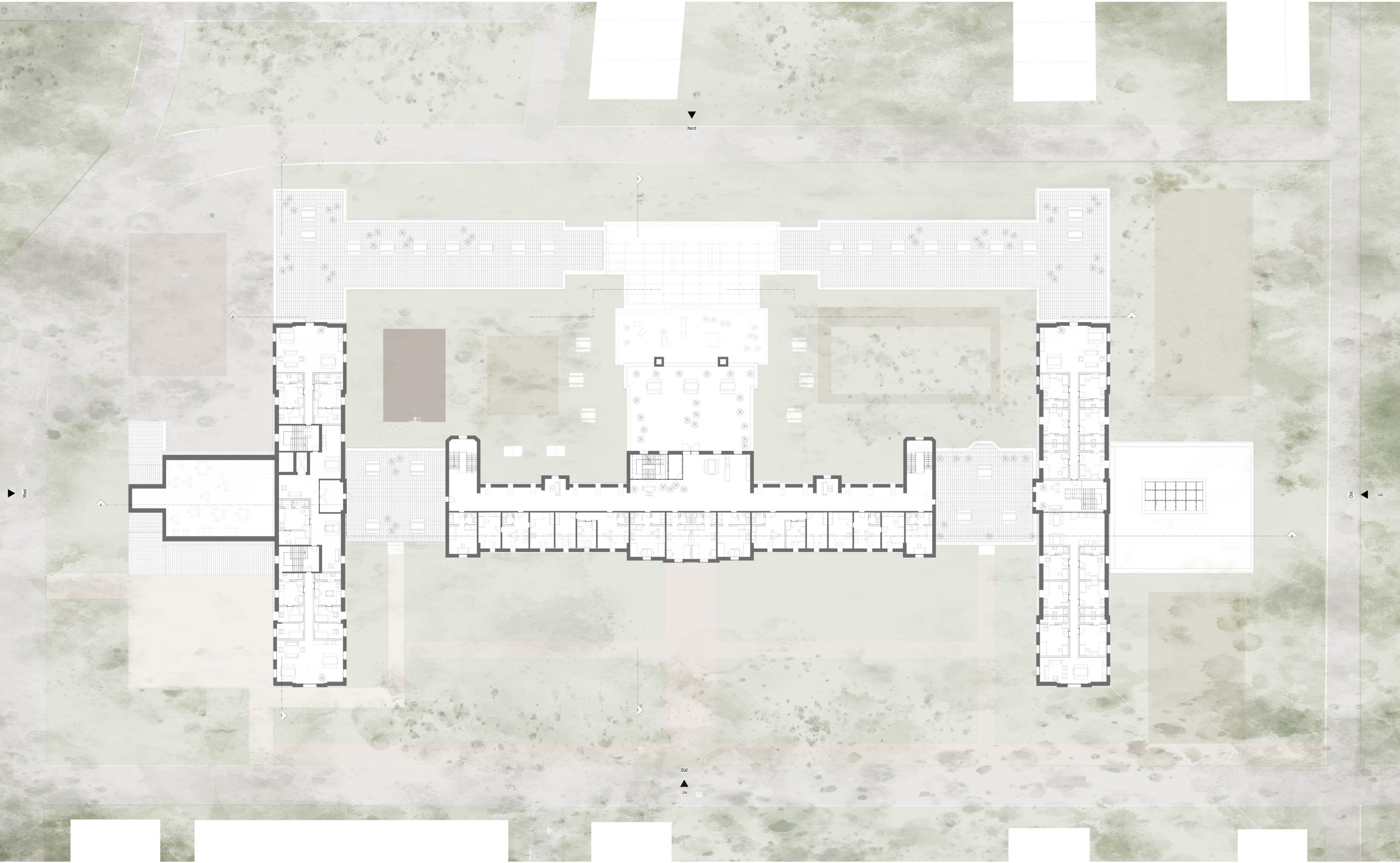
Grundriss 2.OG
