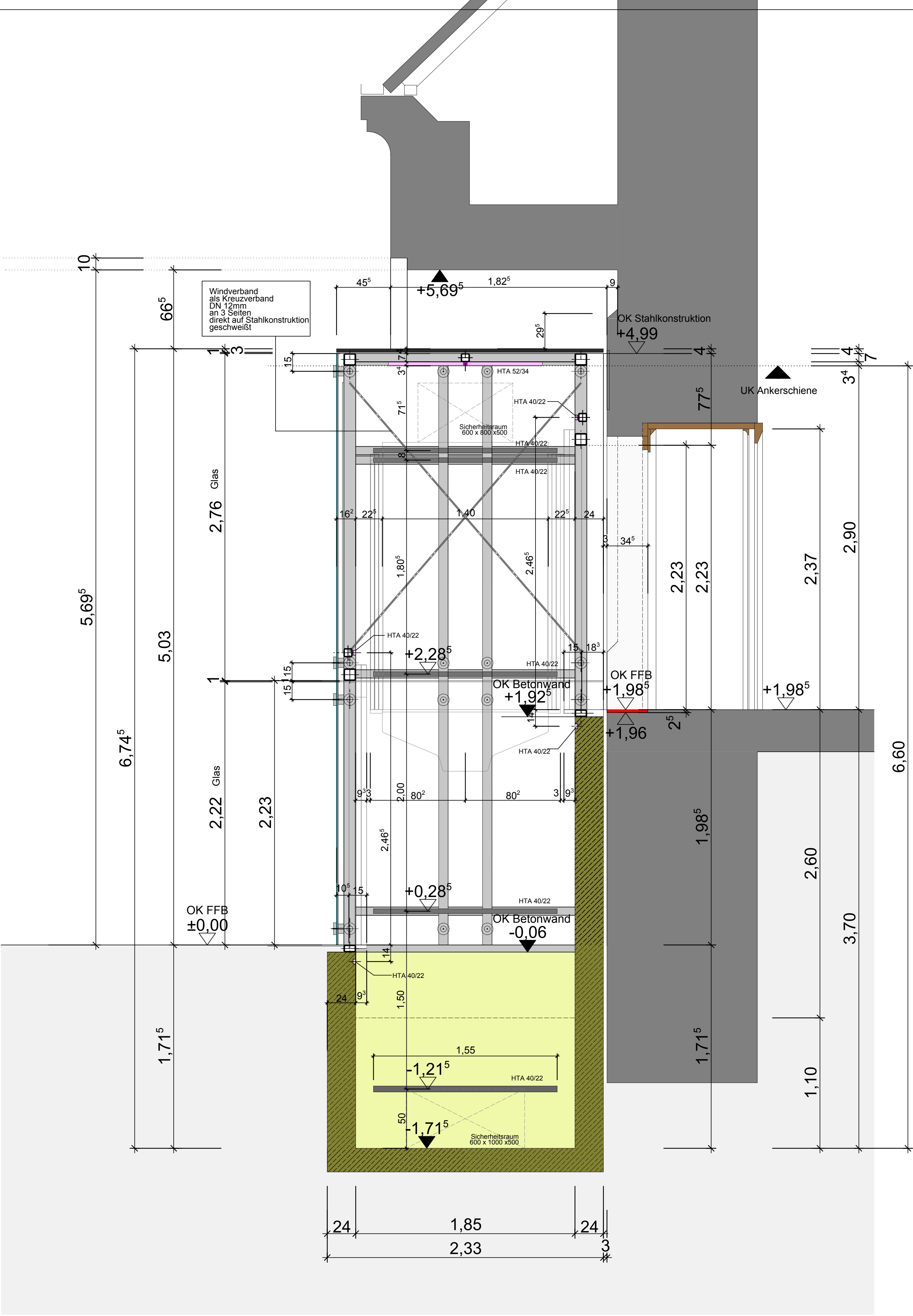
SCHNITT M. 1:20
