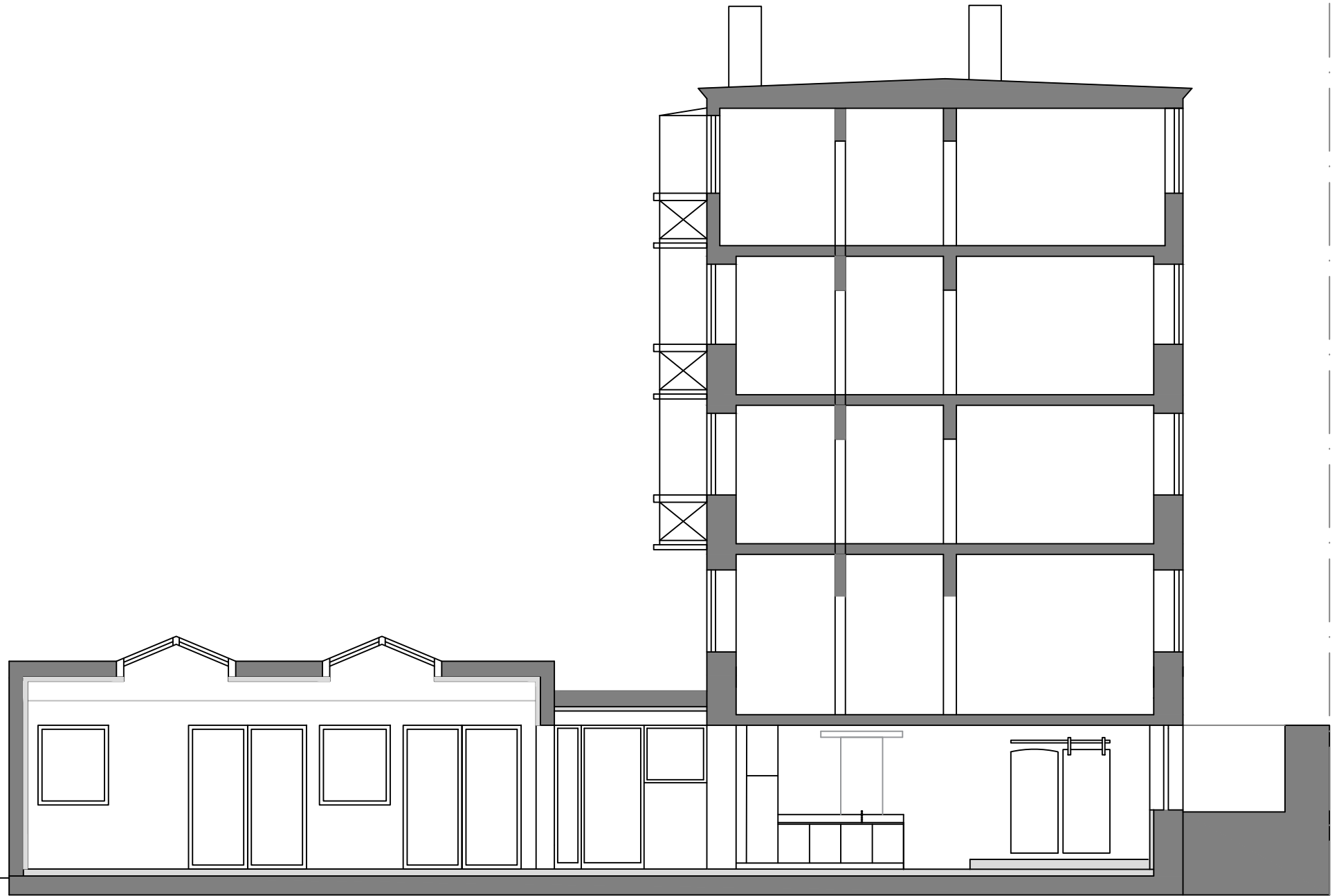
Schnitt C-C
