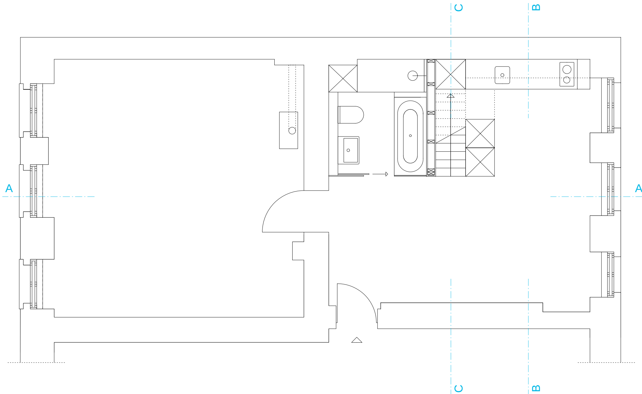
Grundriss EG
