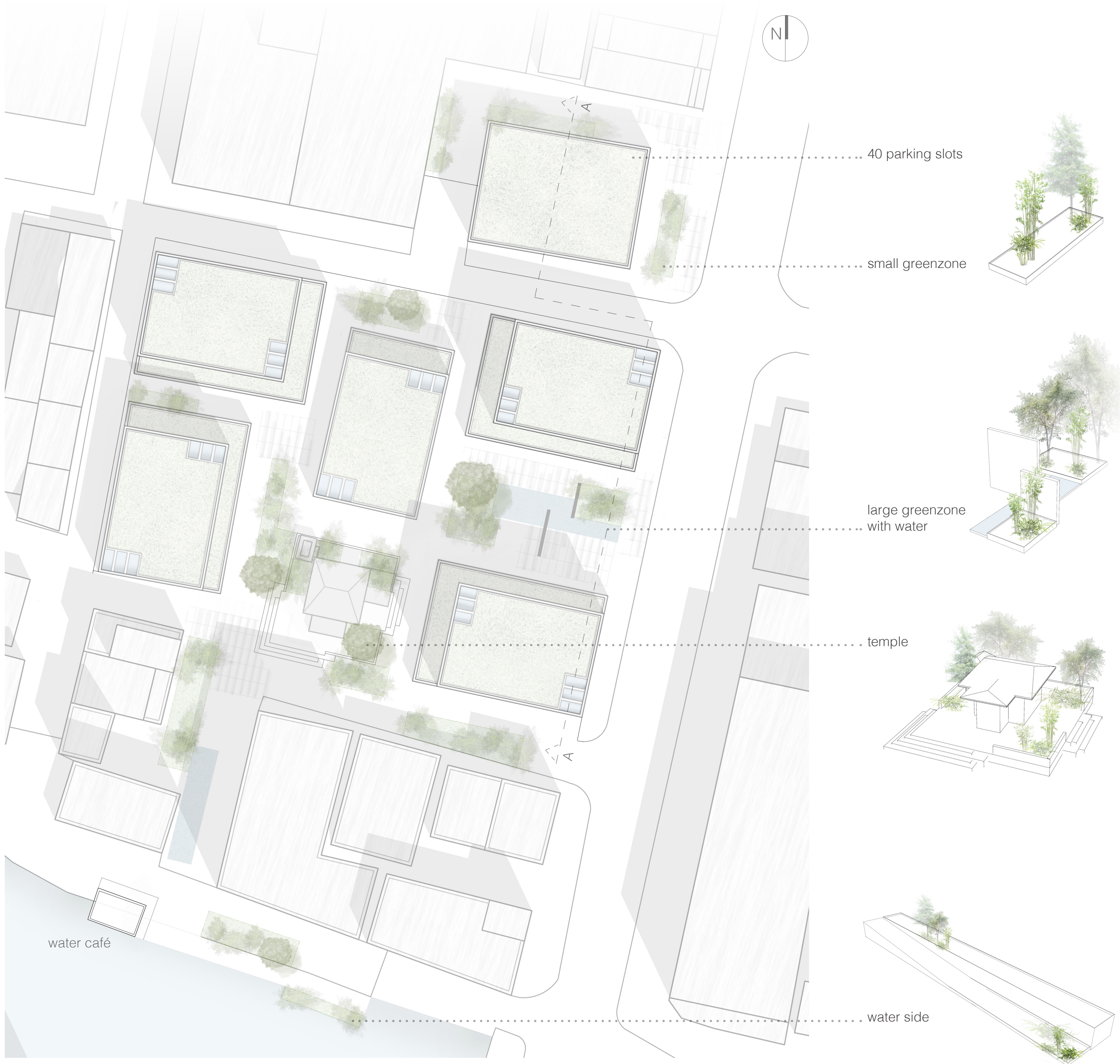
site plan | M 1:250
