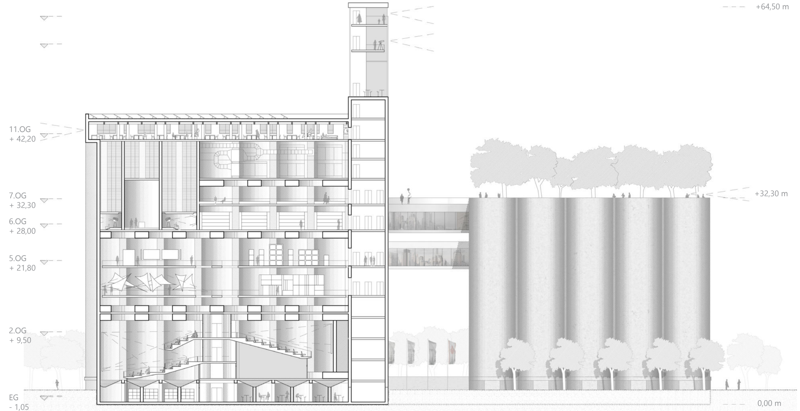
Schnitt A-A u. Ansicht West
