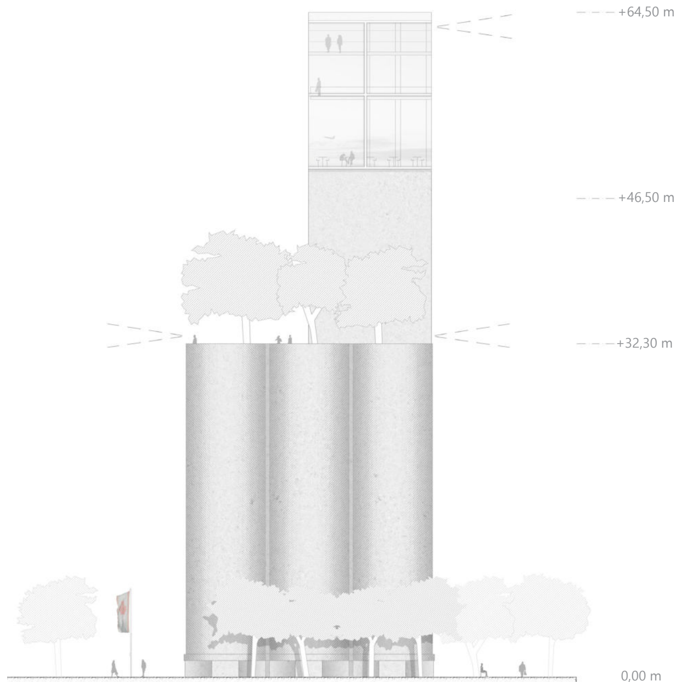
Ansicht Süd
