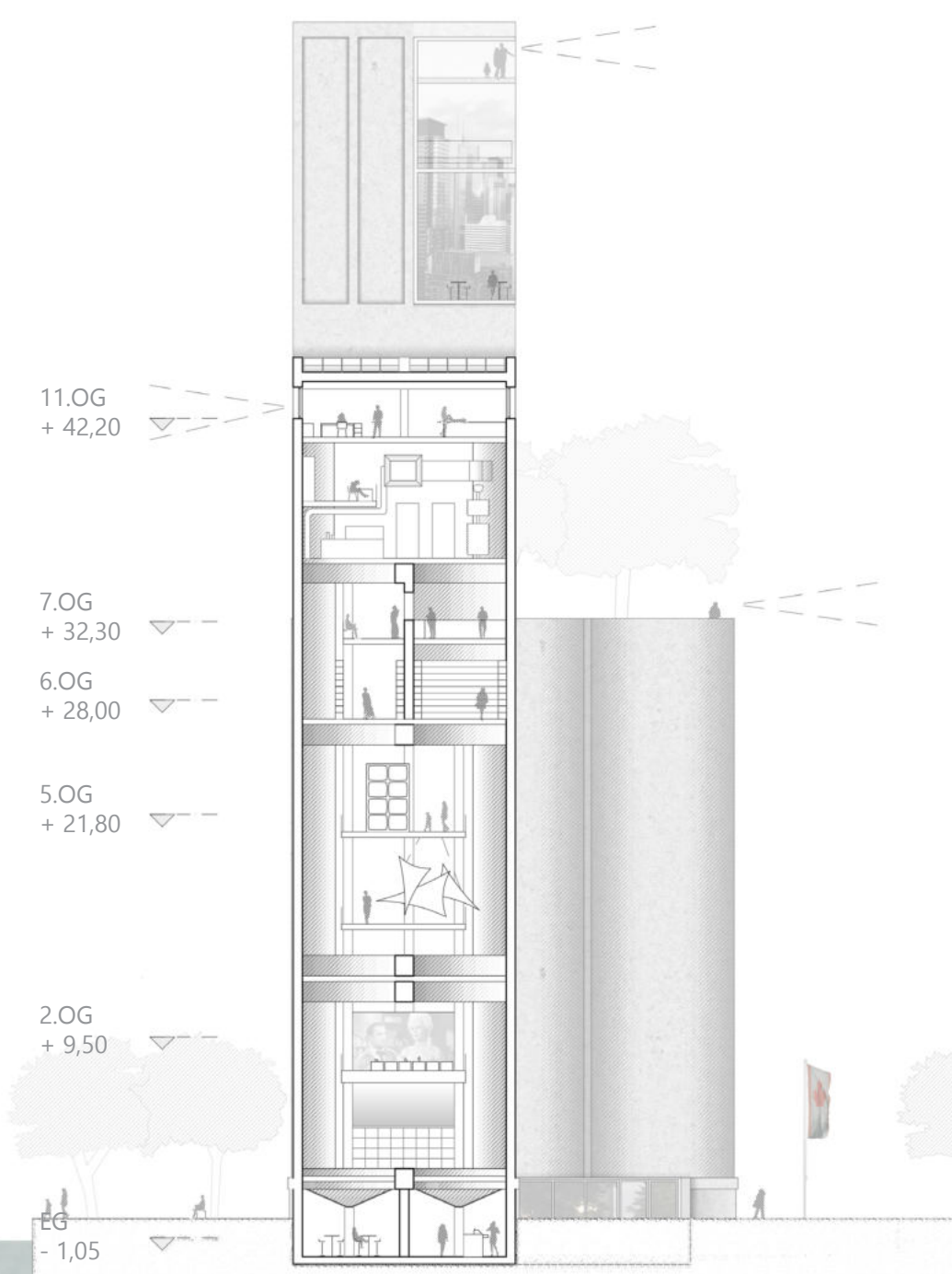
Schnitt D-D & Ansicht Nord
