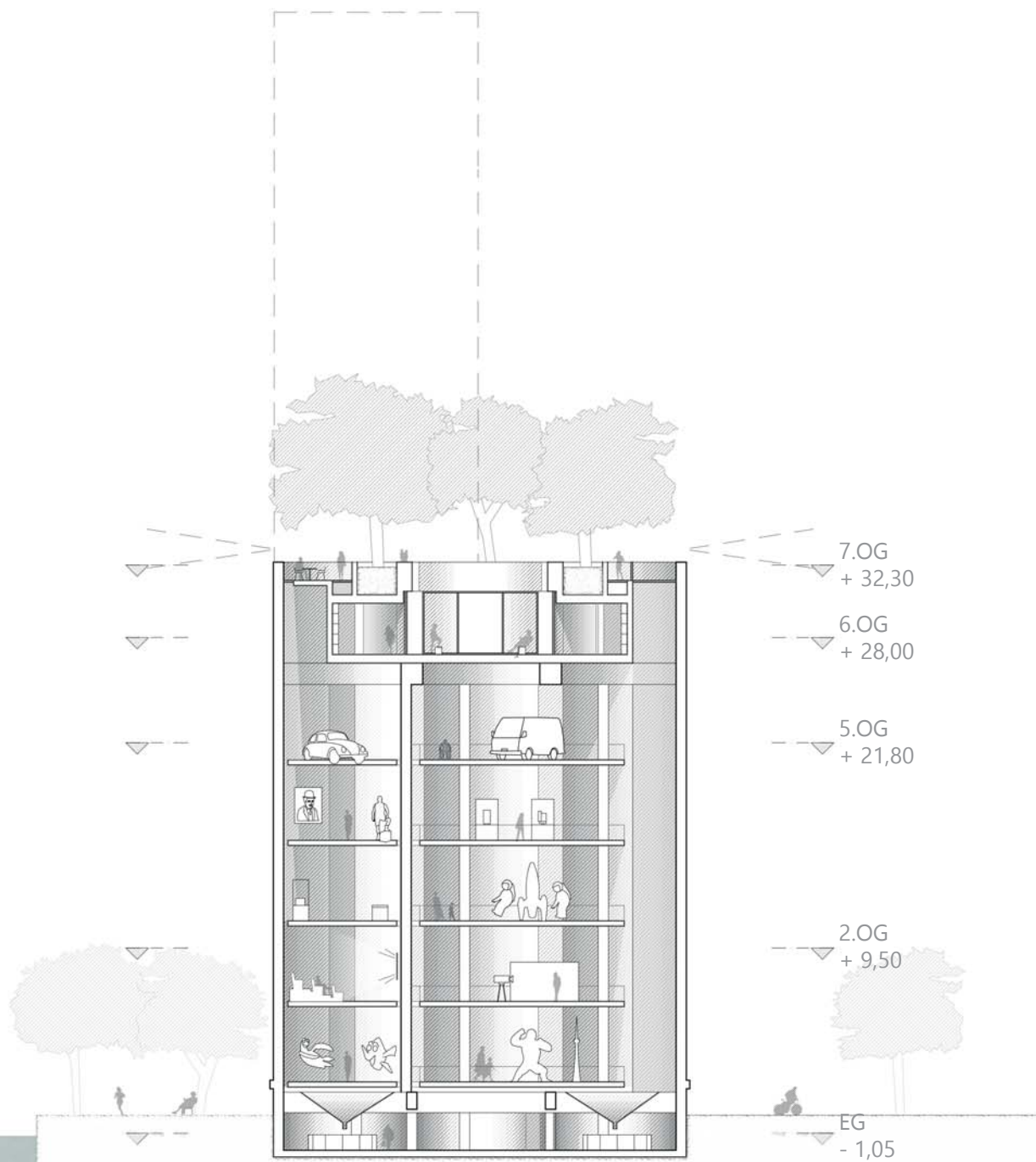
Schnitt C-C
