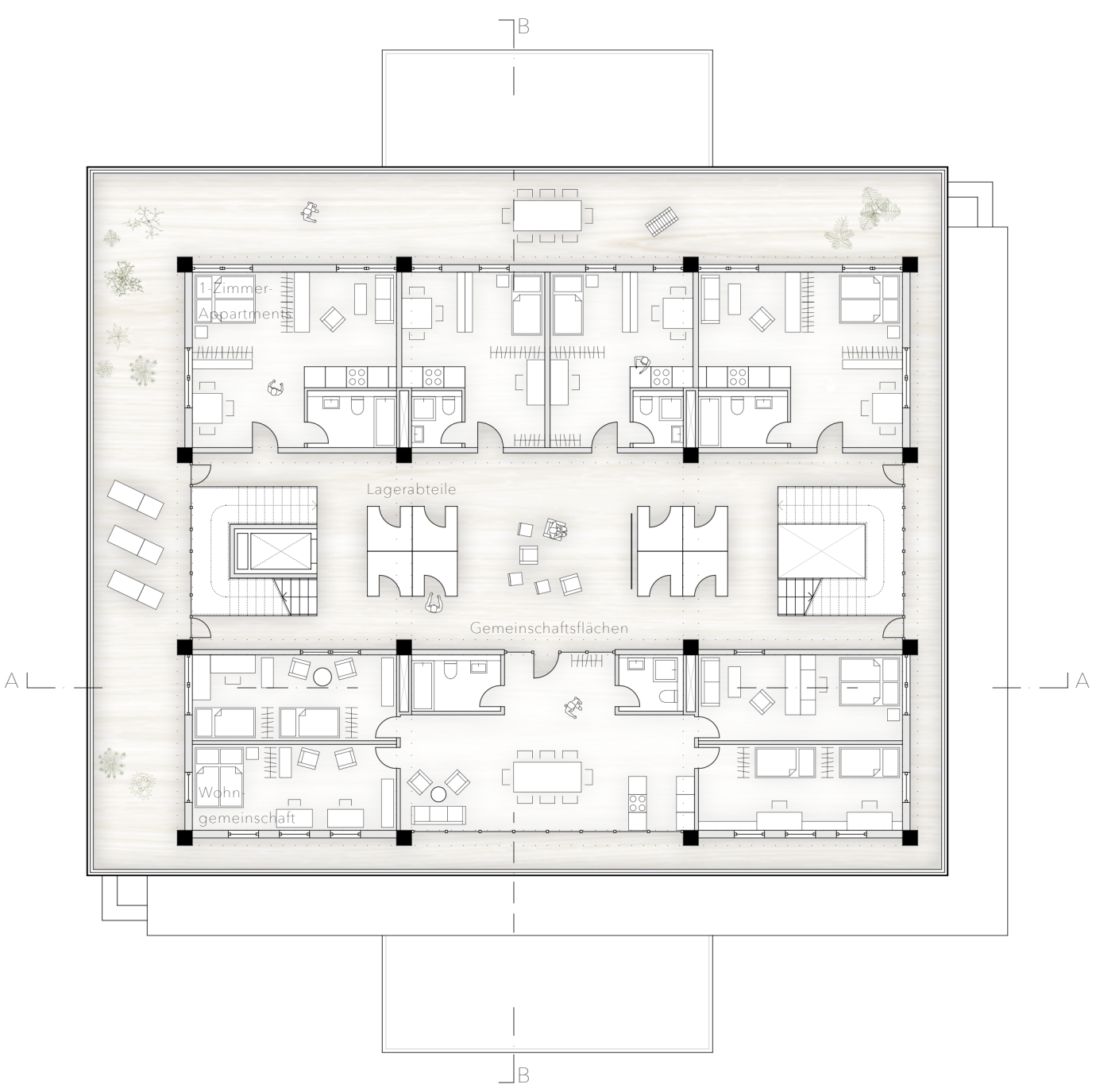
Grundriss OG 6, 8, 10 | 1 : 200
