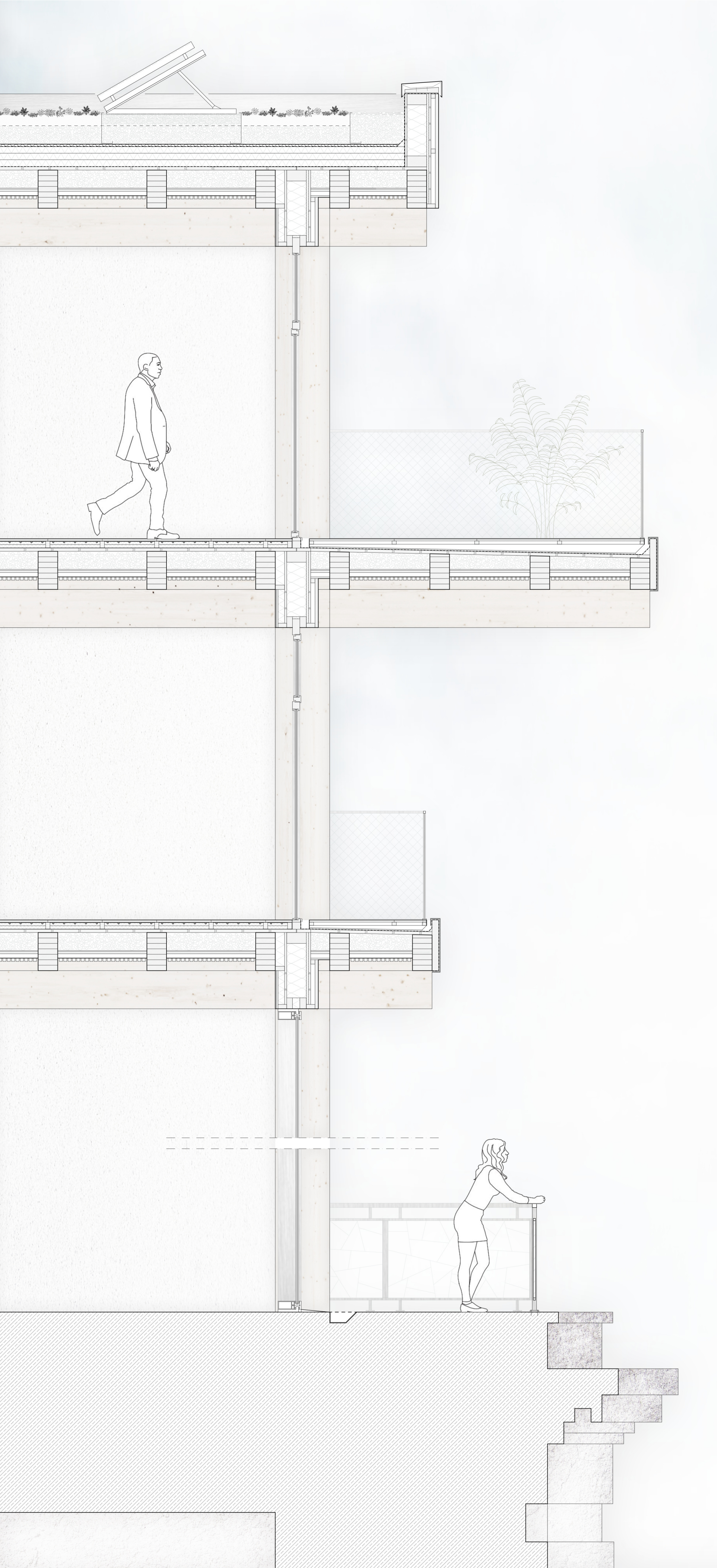
Detailschnitt | 1:20 Konstruktion des Aufsatzes
