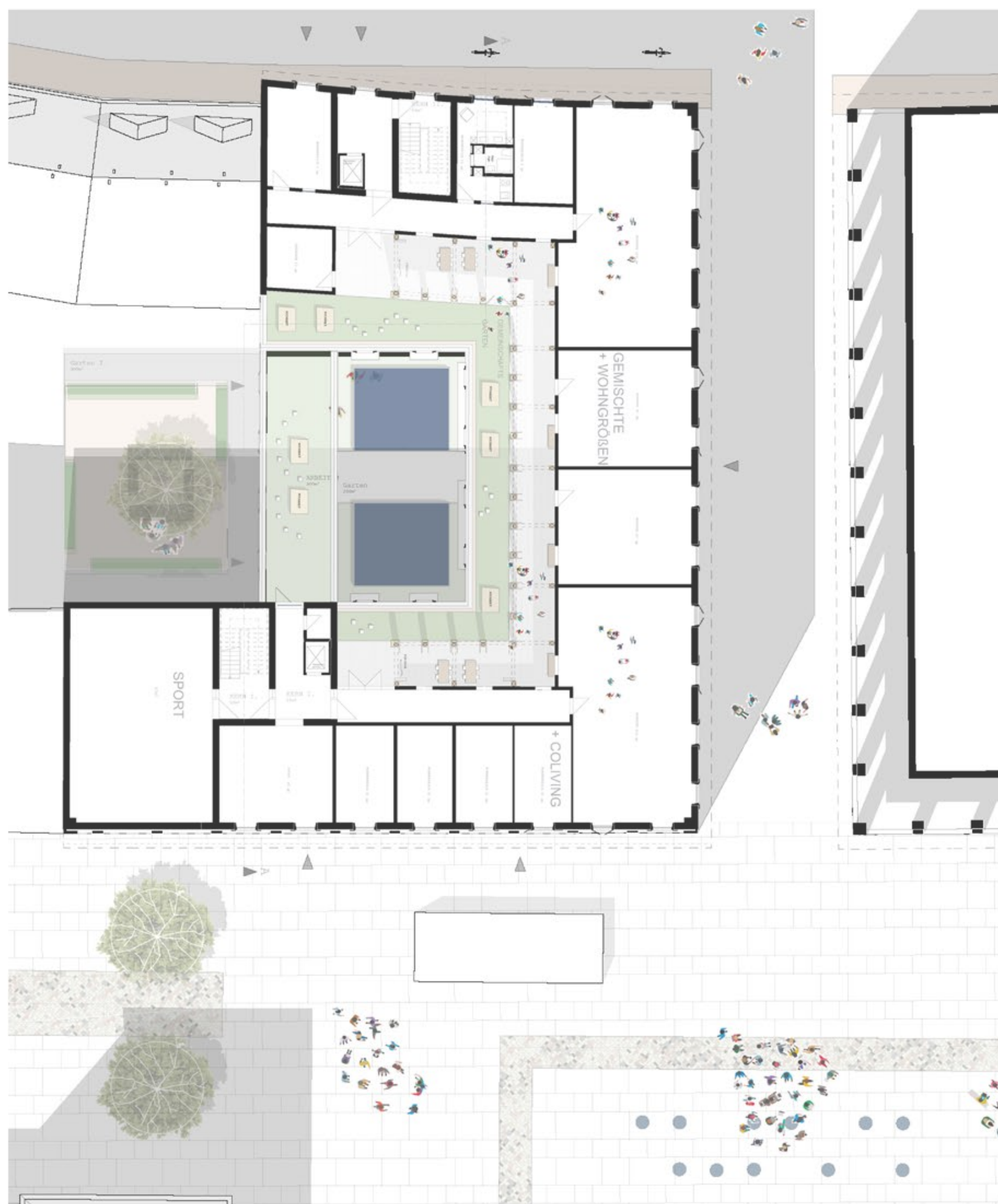
Grundriss EG. M 1:200
