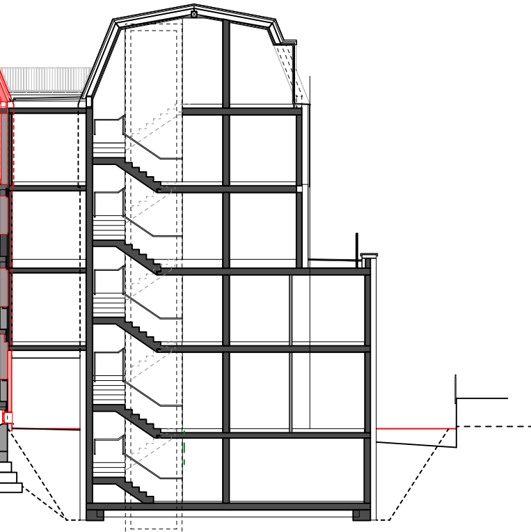
Querschnitt
