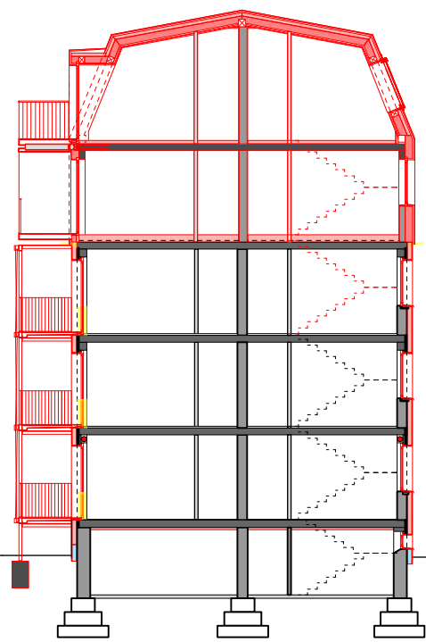
Querschnitt
