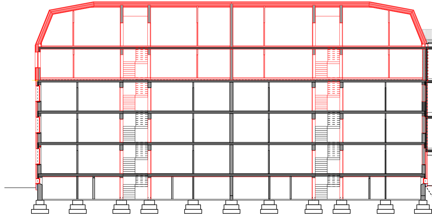
Längsschnitt
