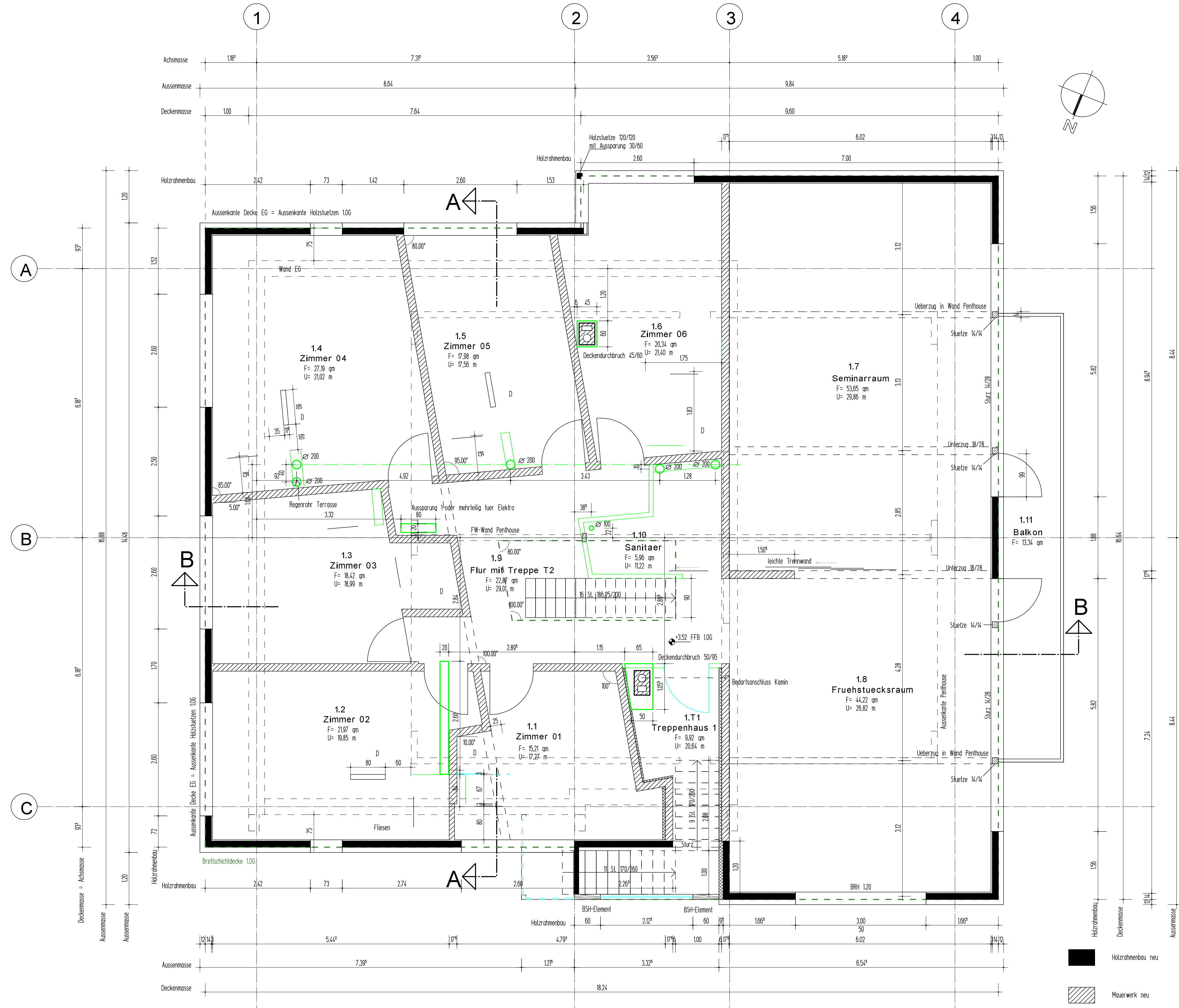
1. Obergeschoss M 1:50
