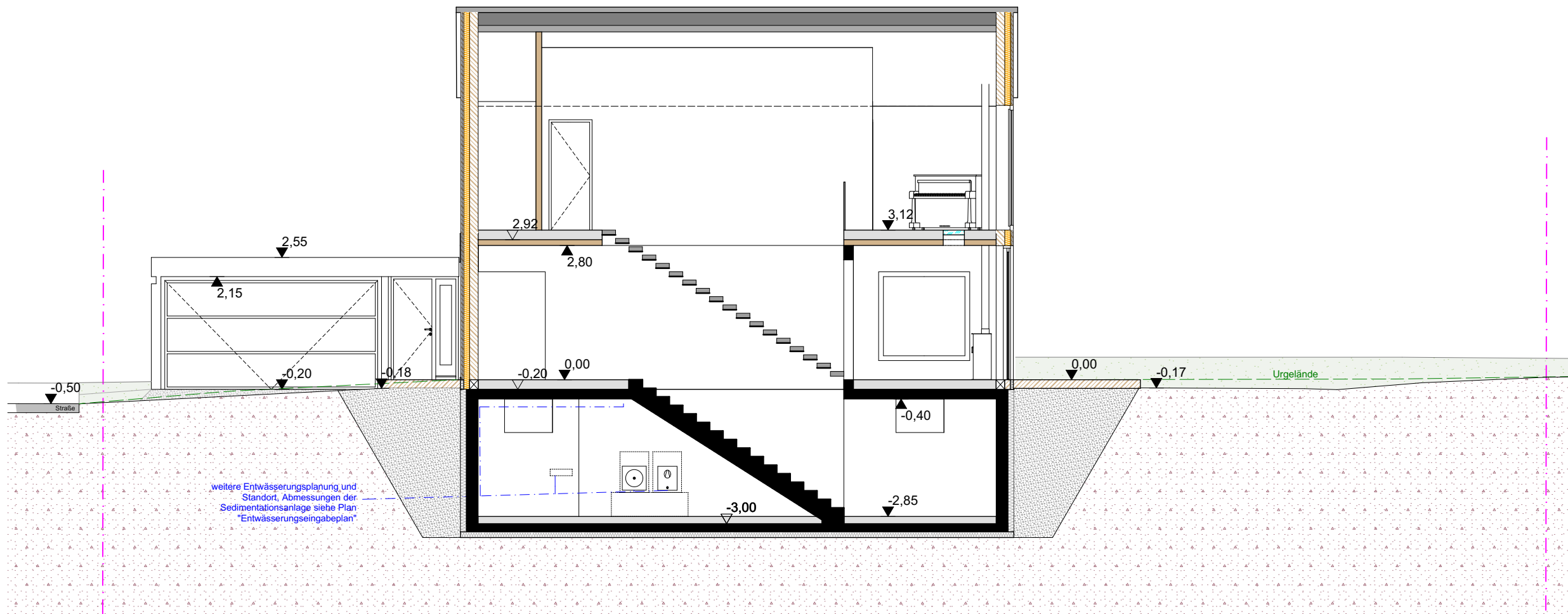
SCHNITT AA
