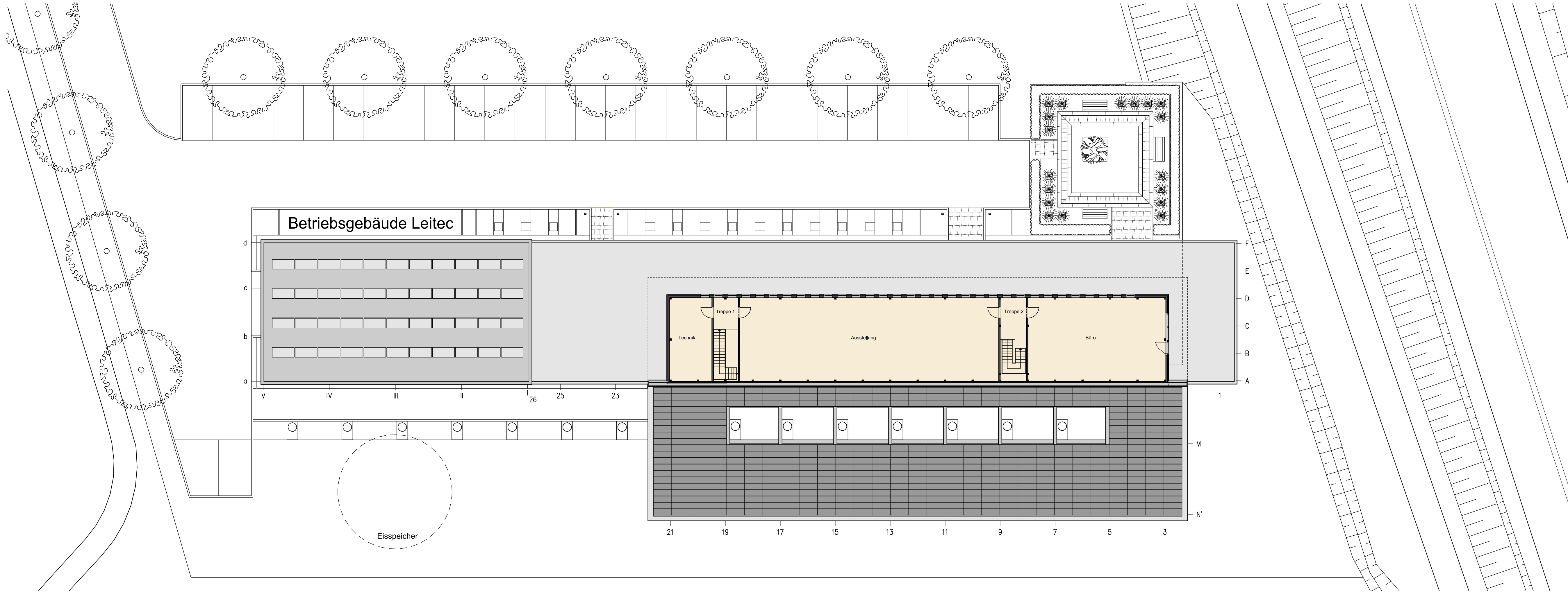
GRUNDRISS OBERGESCHOSS
