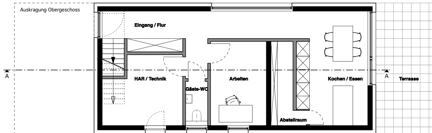
Erdgeschoss
