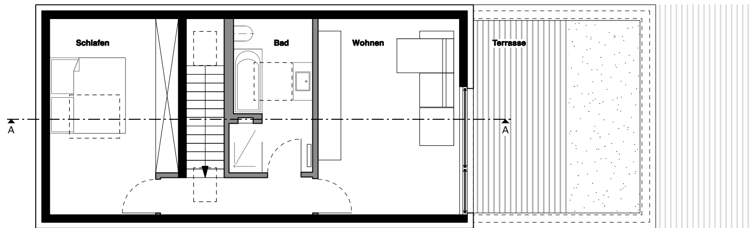
Obergeschoss
