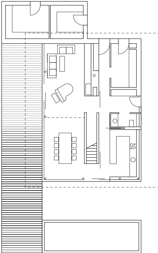
Erdgeschoss
