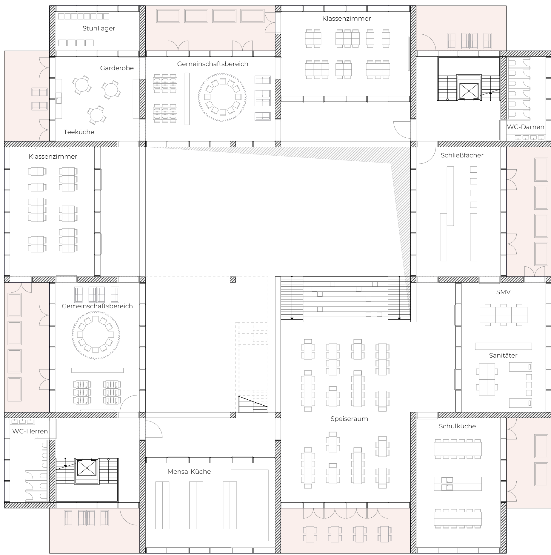
1. OBERGESCHOSS
