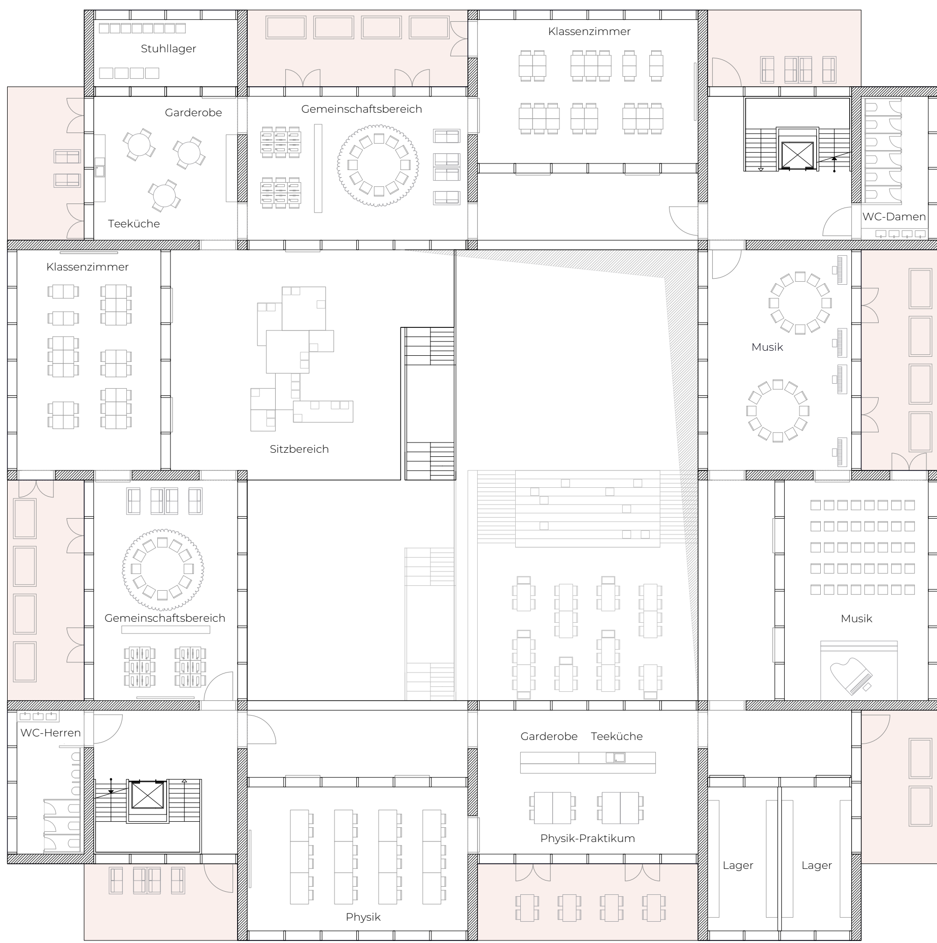
3. OBERGESCHOSS
