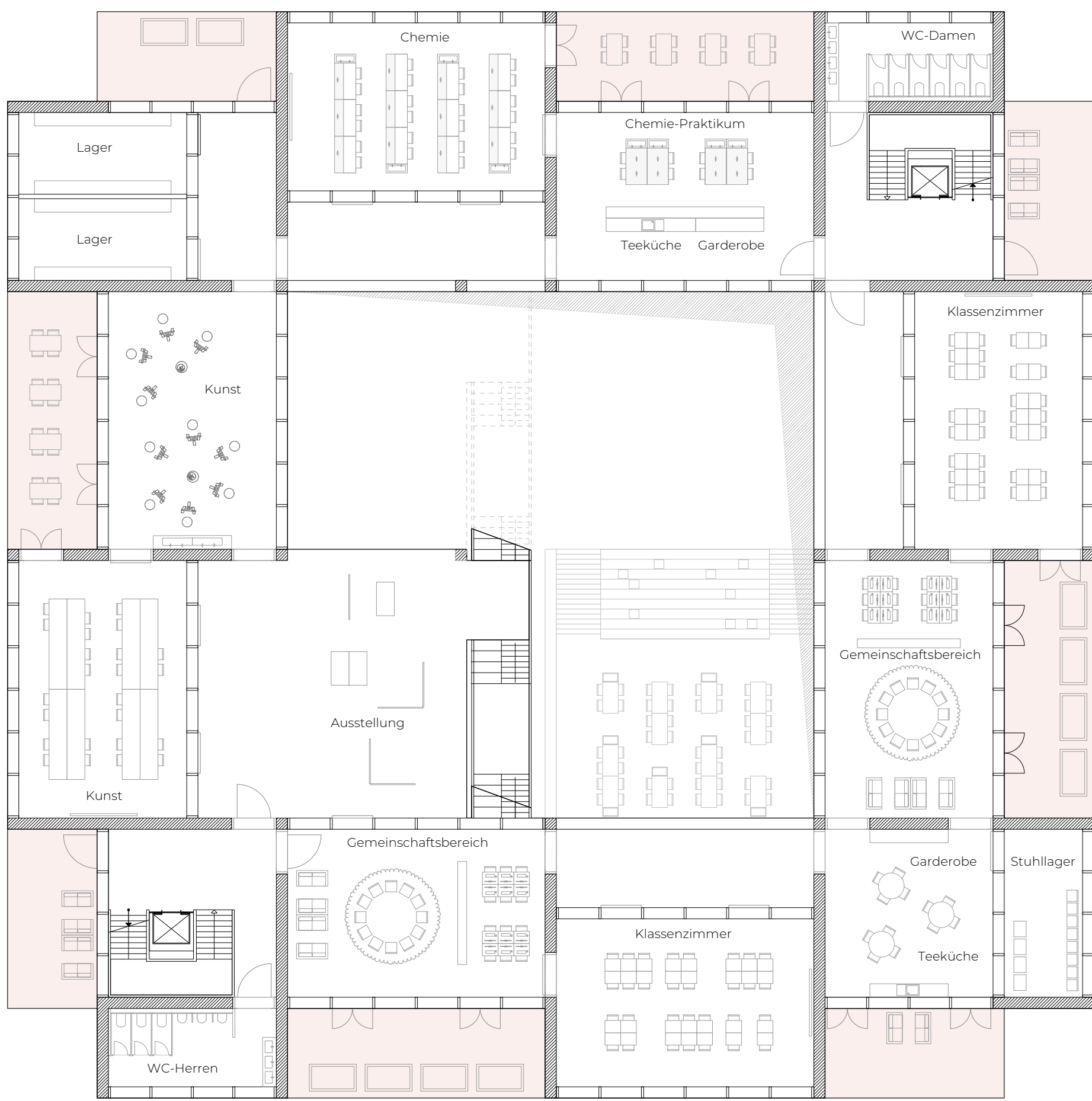
2. OBERGESCHOSS
