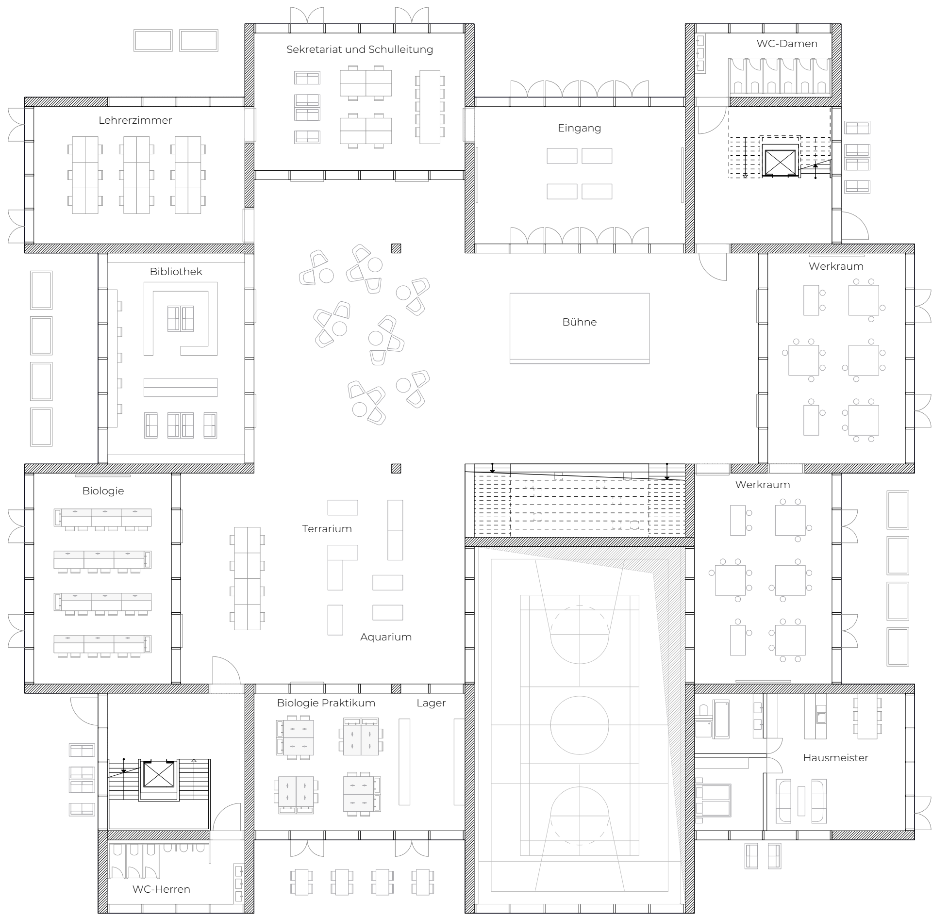
ERDGESCHOSS
